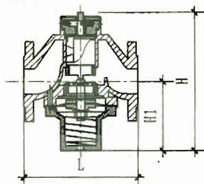
自力式流量控制阀性能与尺寸表
