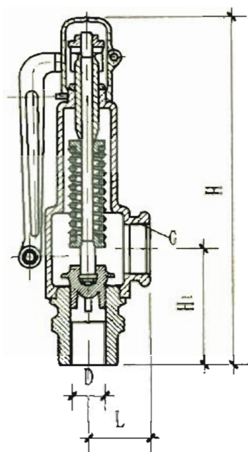
A27W-10型弹簧安全阀
