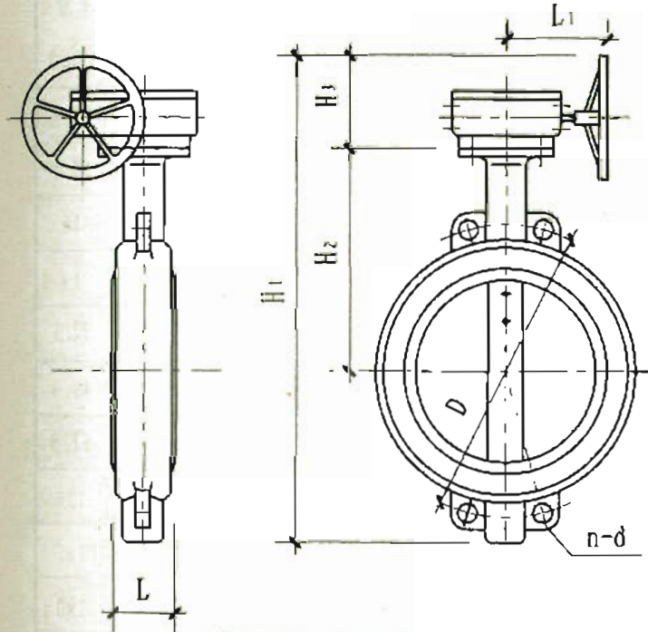
D371X (H、F) 型蜗轮传动对夹式蝶阀 (DN150~700)
