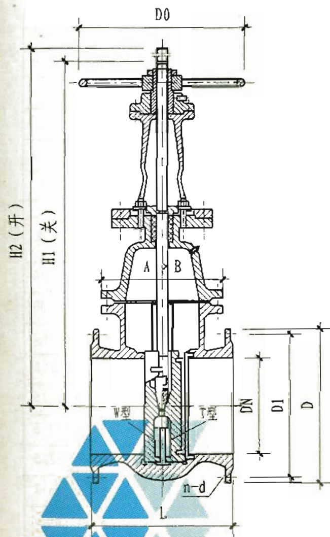
Z44 T W -10型平行式双闸板闸阀
