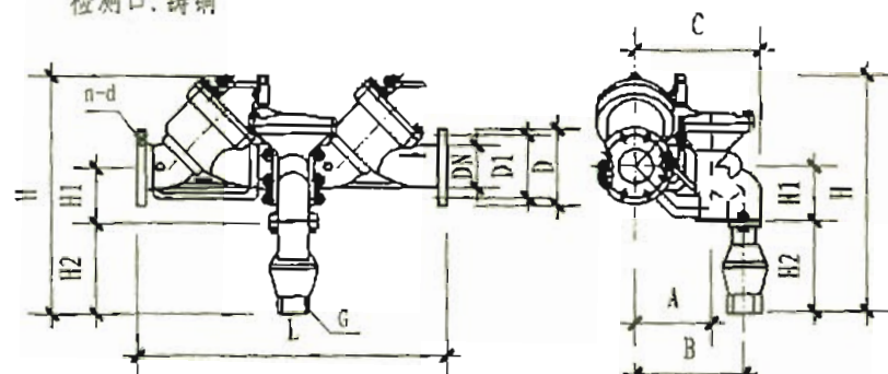
倒流防止器 WT-F909
