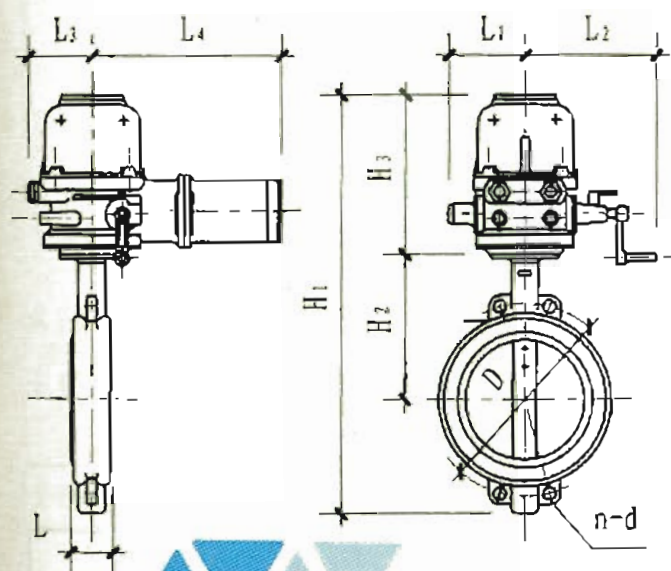
PD971F-25Q电动偏心式蝶阀
