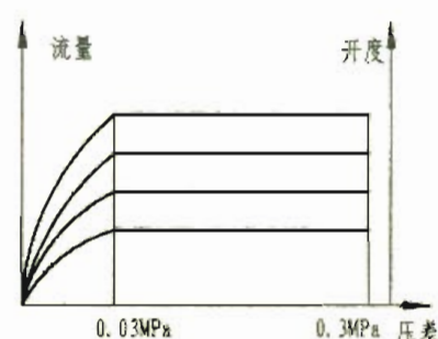
流量-压差曲线
