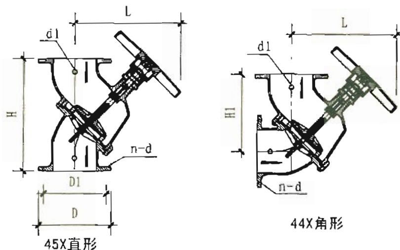
W-JH45/44X四功能泵控阀外形尺寸 (mm)
