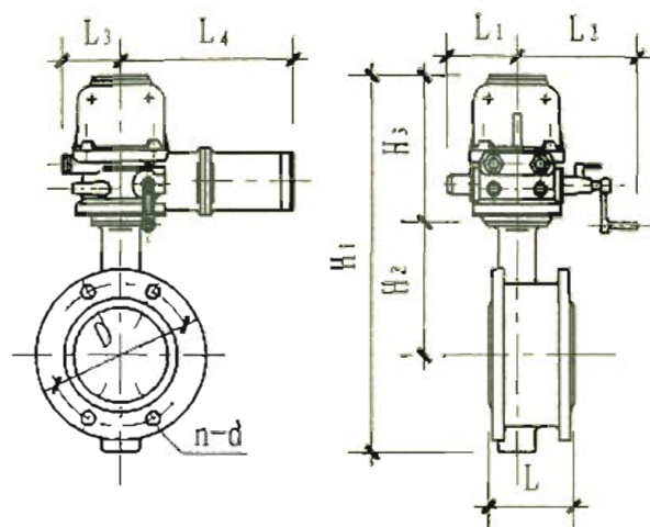
D941型电动法兰式蝶阀 (DN80~700)
