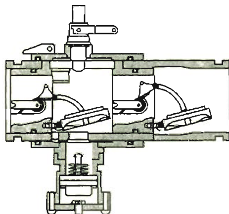
倒流防止器 WT-957
