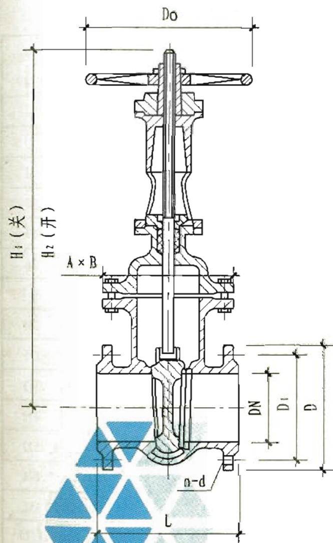
Z41T-10型明杆楔式闸阀
