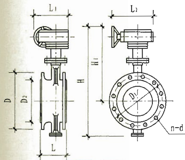
D343H型法兰式三偏心硬密封蝶阀
