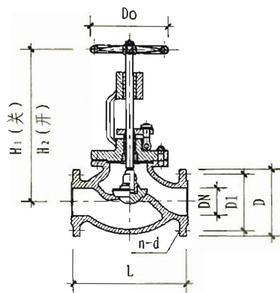
J41H型手动截止阀
