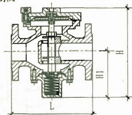
自力式压差控制阀性能与尺寸表
