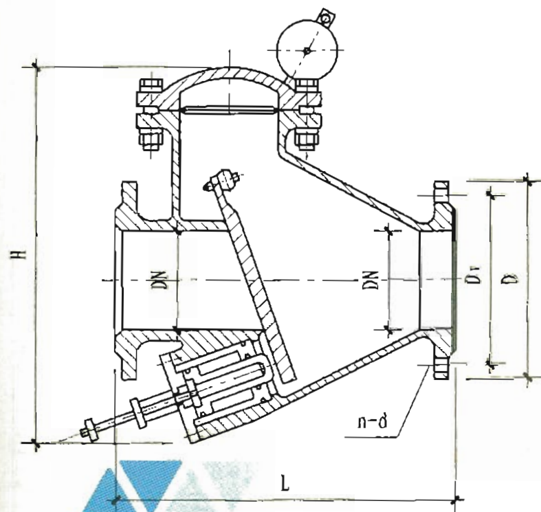
HH44X- \frac{10}{16} 型微阻缓闭止回阀
