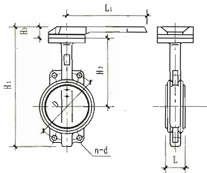
D71X型手柄传动对夹式蝶阀
