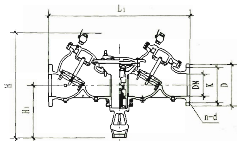
(不带过滤) 倒流防止器 (法兰型)
