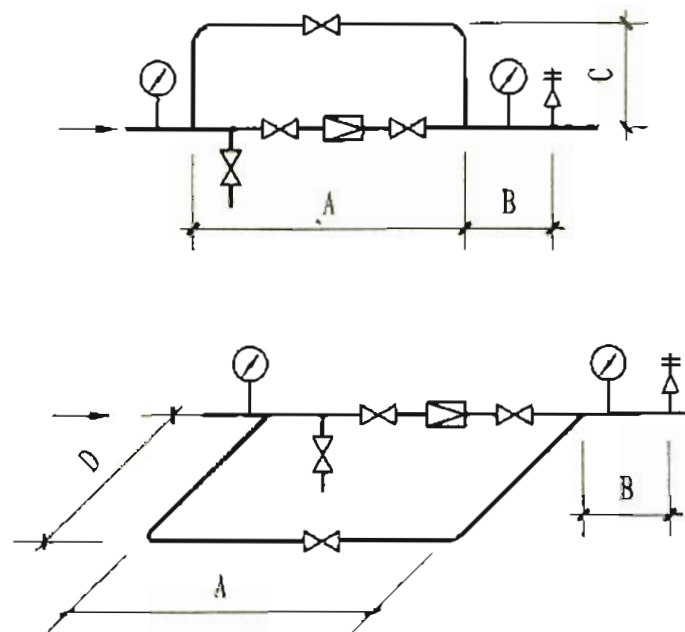
活塞式减压阀安装示意图
