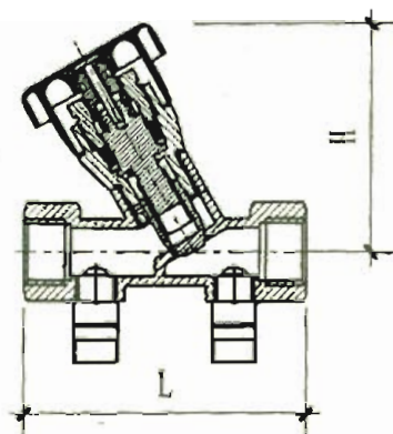
丝扣连接静态水力平衡阀
