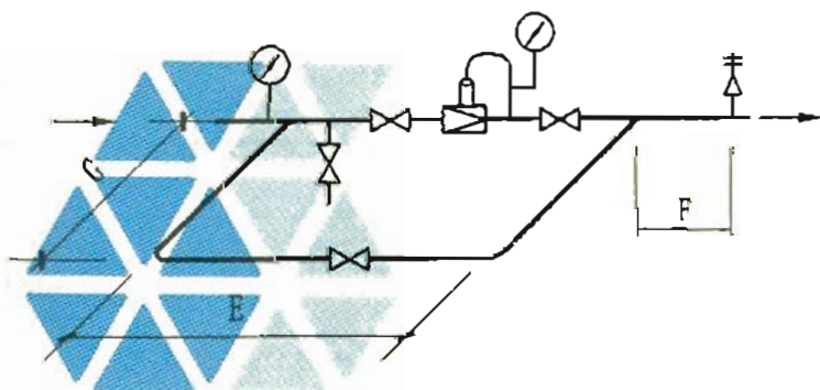
薄膜式（波纹管式）减压阀安装示意图
