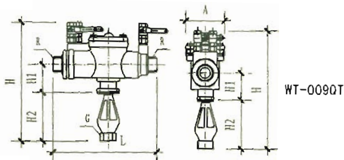
倒流防止器 WT-009QT尺寸表 (mm)
