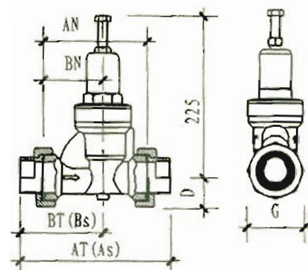
N45B 型供水减压阀尺寸表 (mm)
