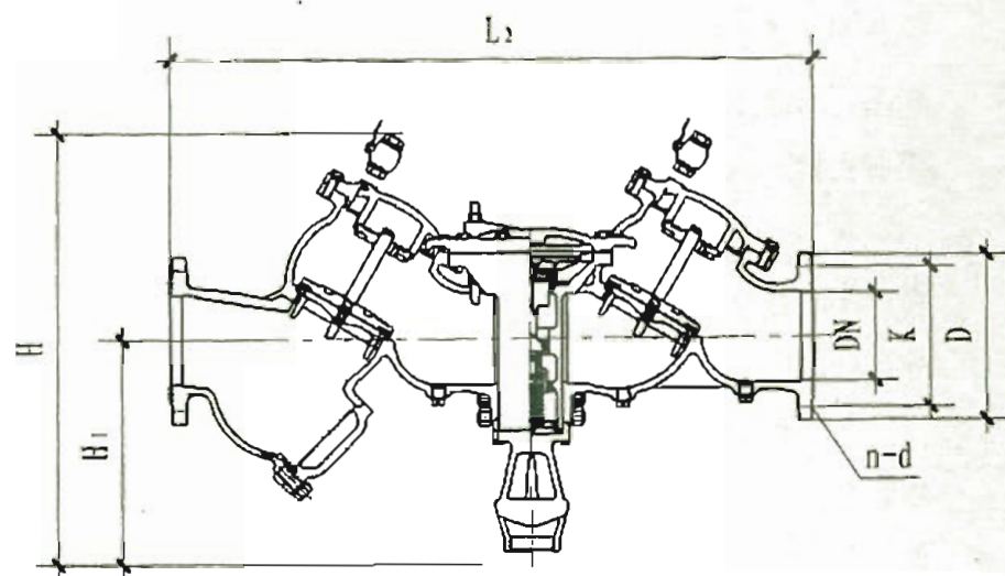
(带过滤) 倒流防止器 (法兰型)
