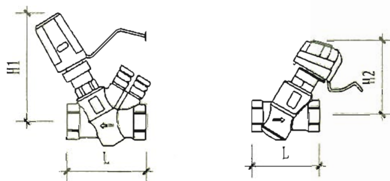
EV. 0.3/ EV. 0.4 执行器, A阀体
