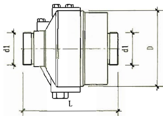
W-TZCY11-16Q型 (DN15-DN32)
