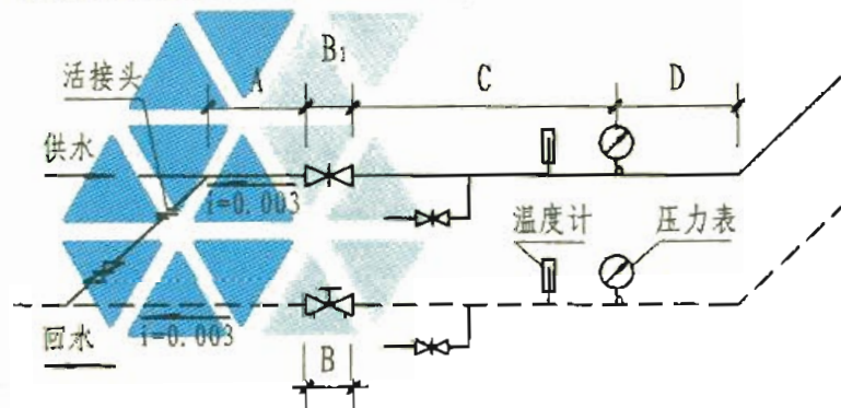
平衡阀在热力入口的安装
