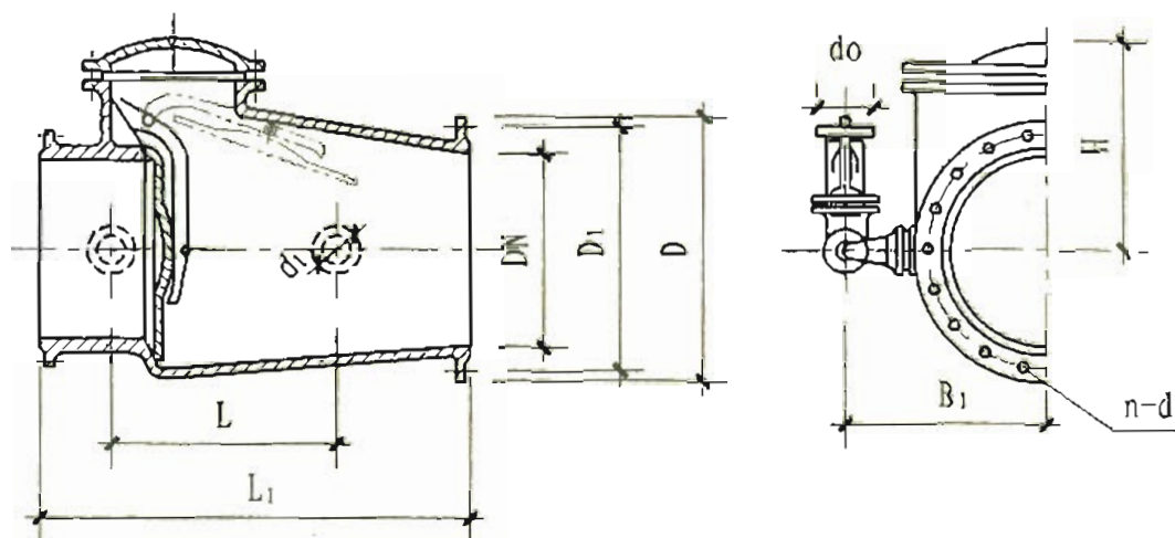
H44T(X)-10型旋启式止回阀
