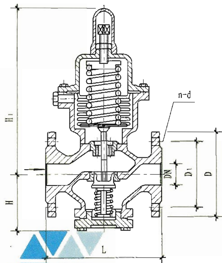
Y44T-10型波纹管式减压阀
