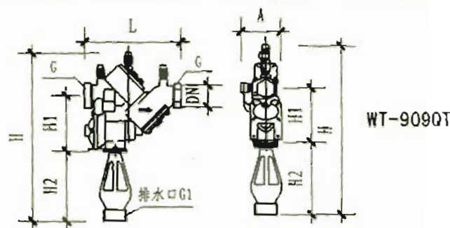
倒流防止器 WT-909QT尺寸表 (mm)
