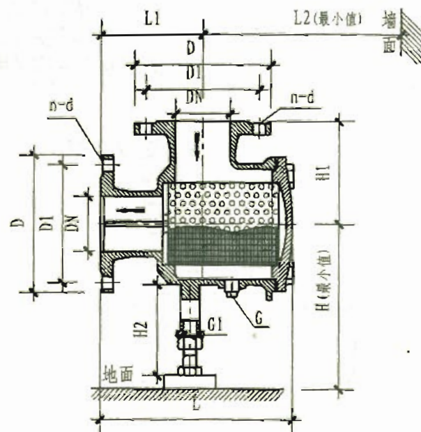
W-JZG44角形整流过滤器外形尺寸 (mm)
