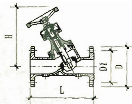
法兰连接静态水力平衡阀
