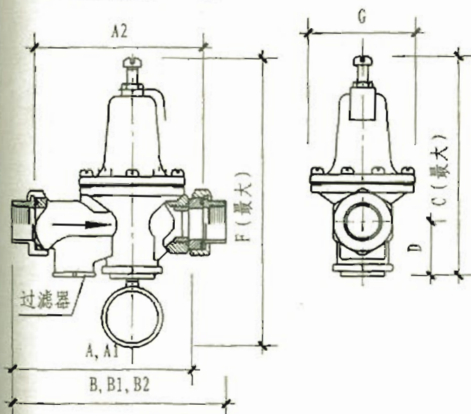
25AUB型供水减压阀尺寸表 (mm)
