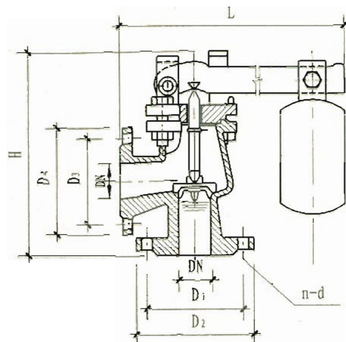
单杆微启式安全阀
