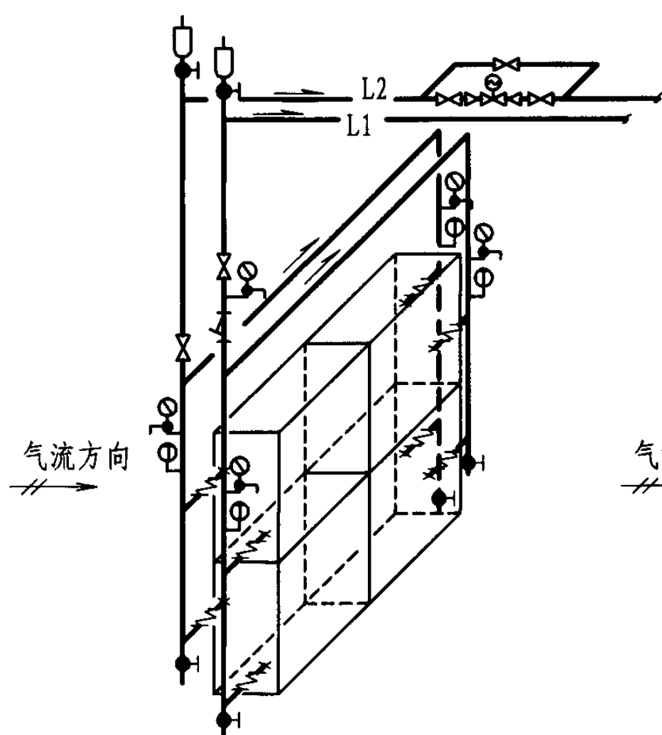
四台冷却器接管示意图
