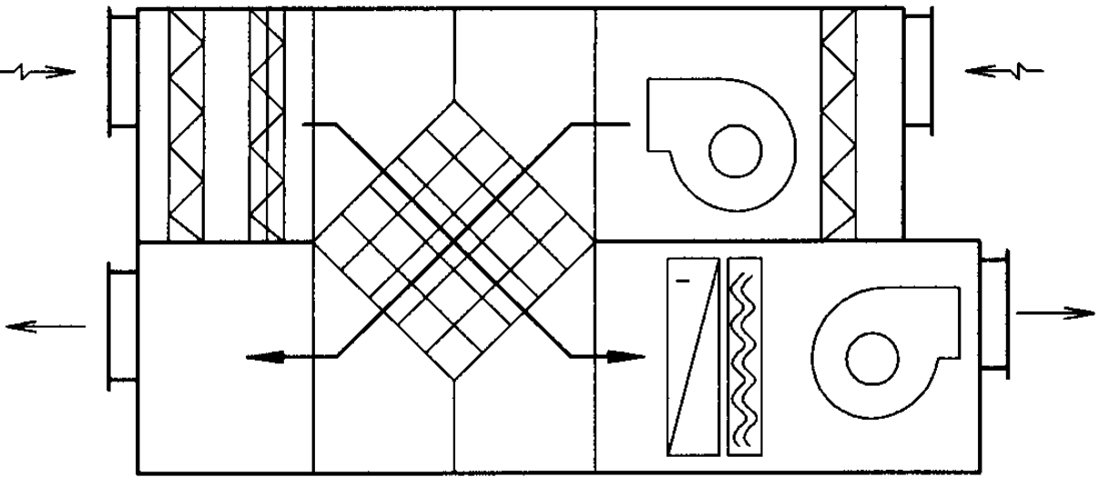
板式能量回收空气处理机组
