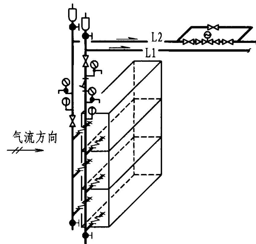
三台冷却器接管示意图
