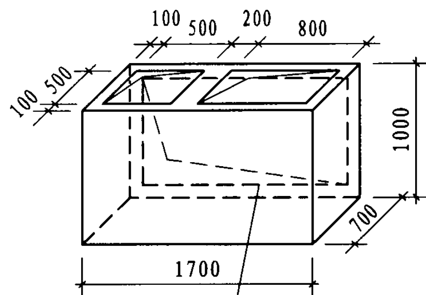
联箱详图
