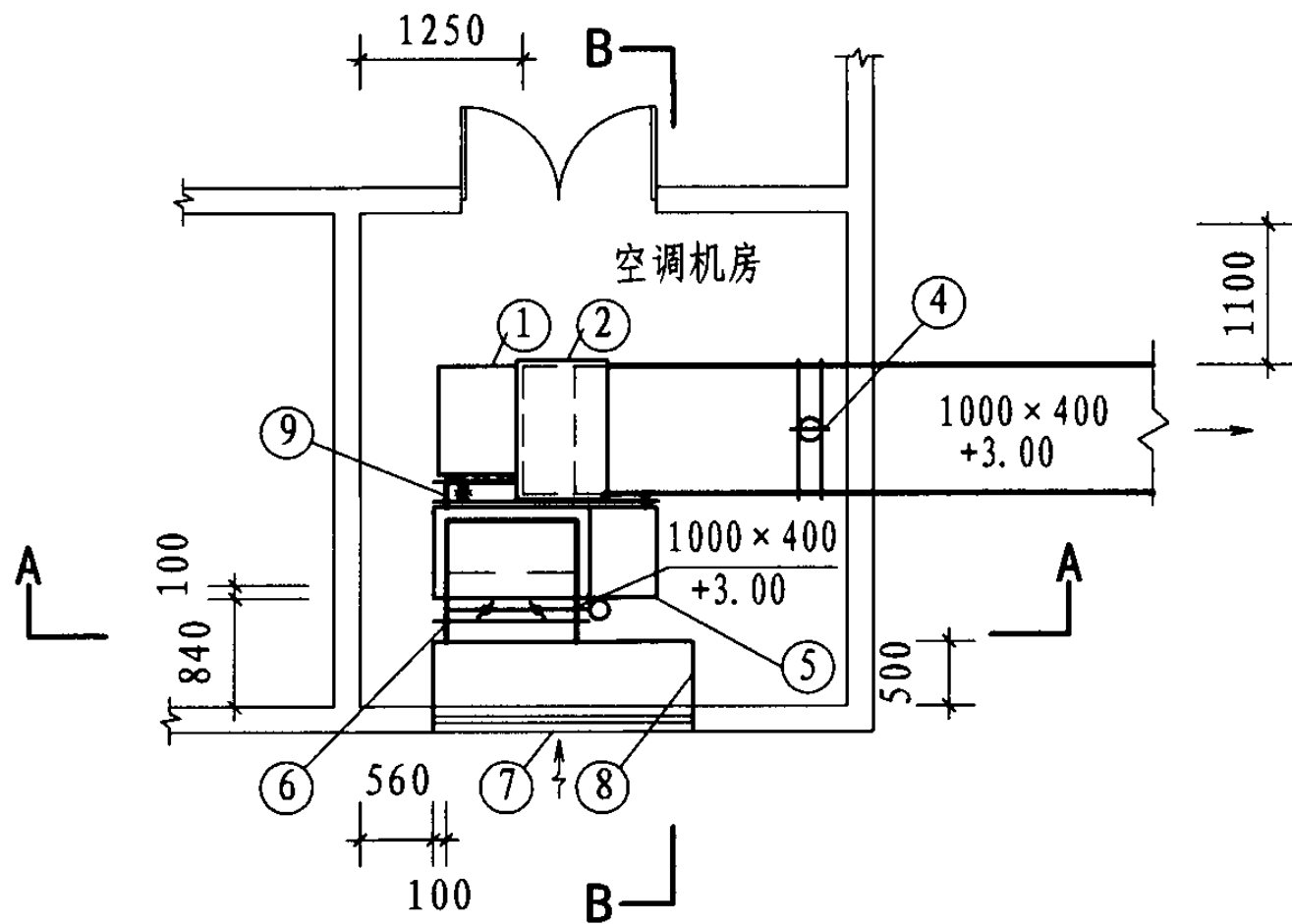
风管平面图
