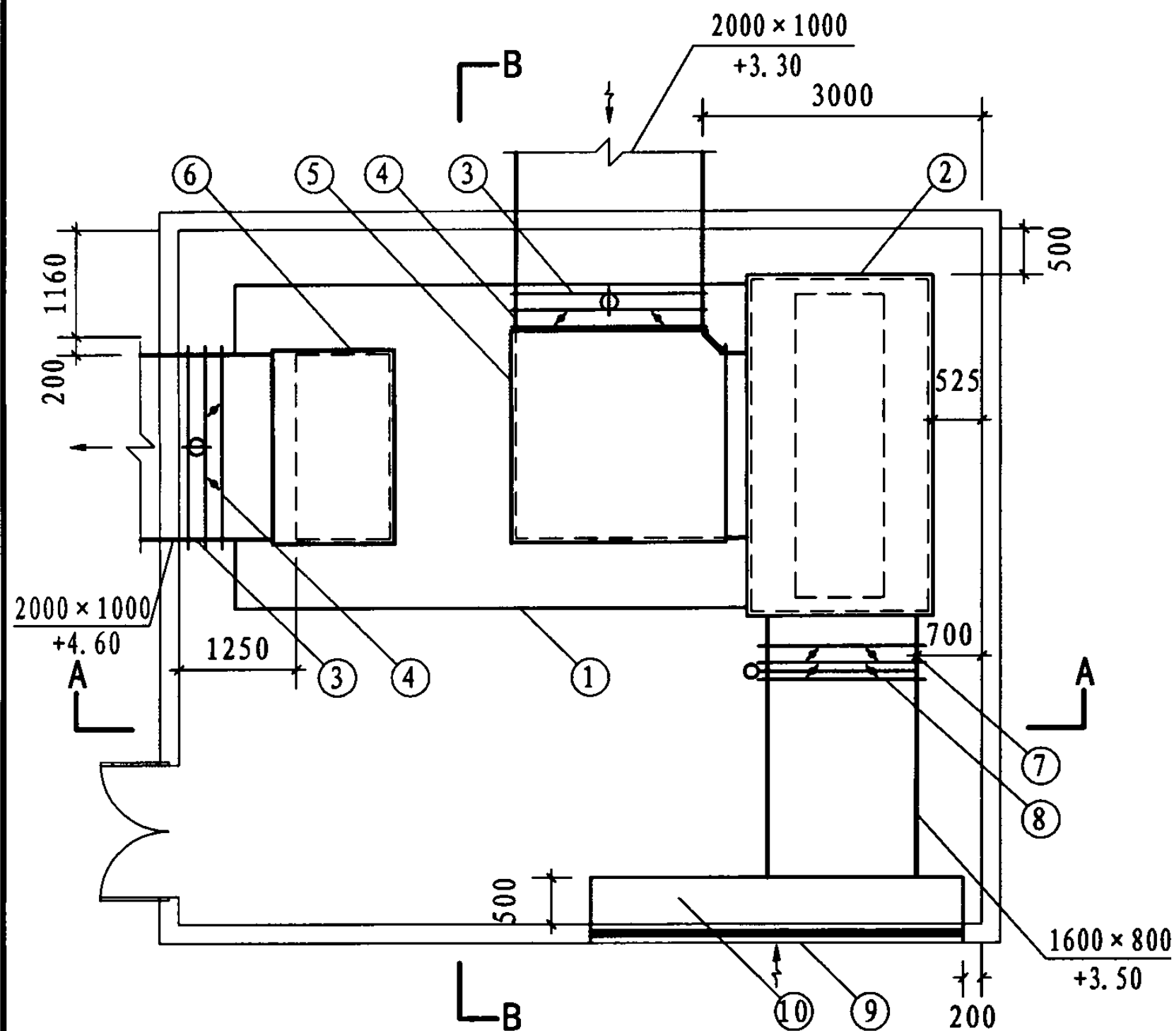
风管平面图
