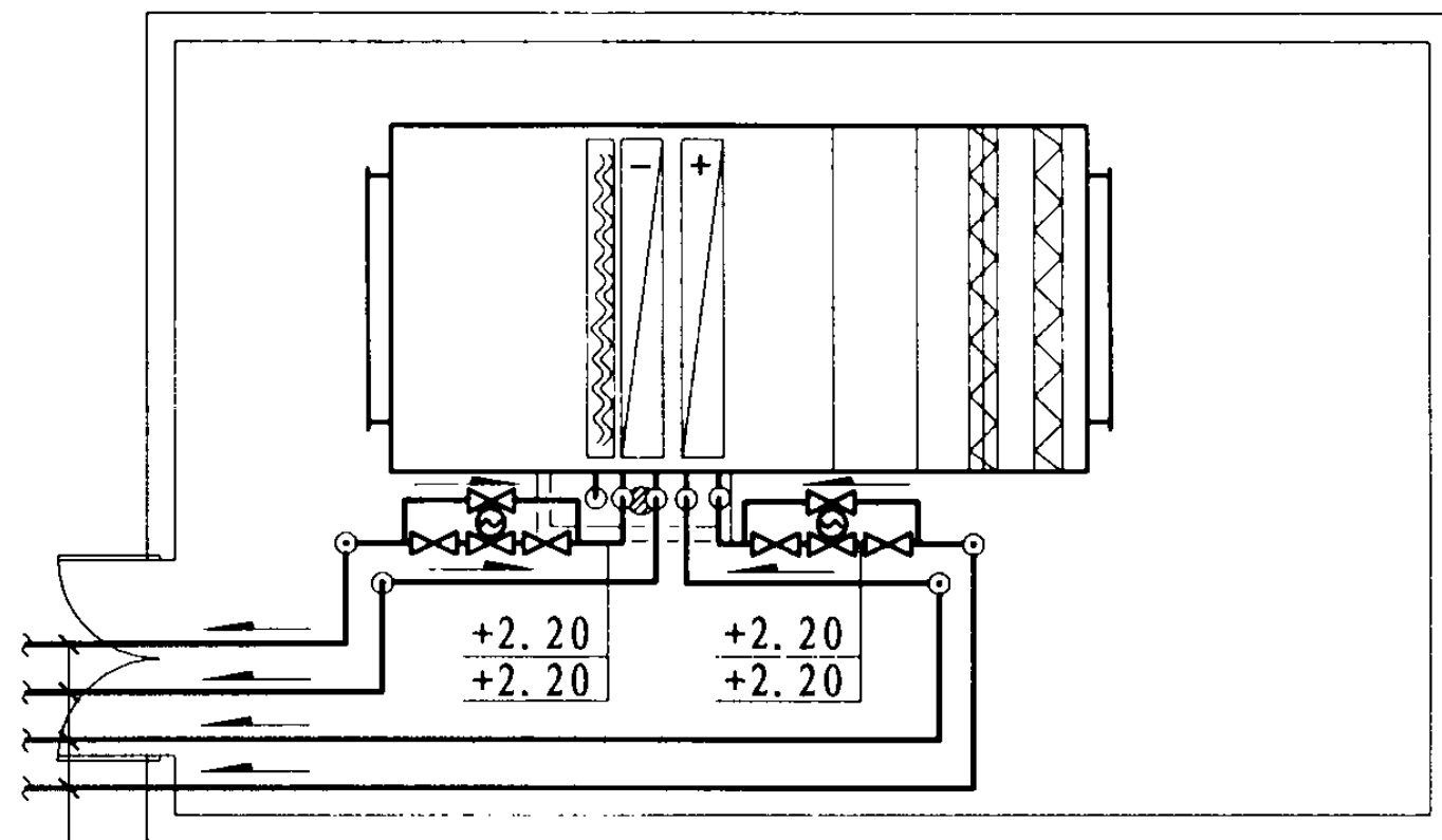
水管平面图
