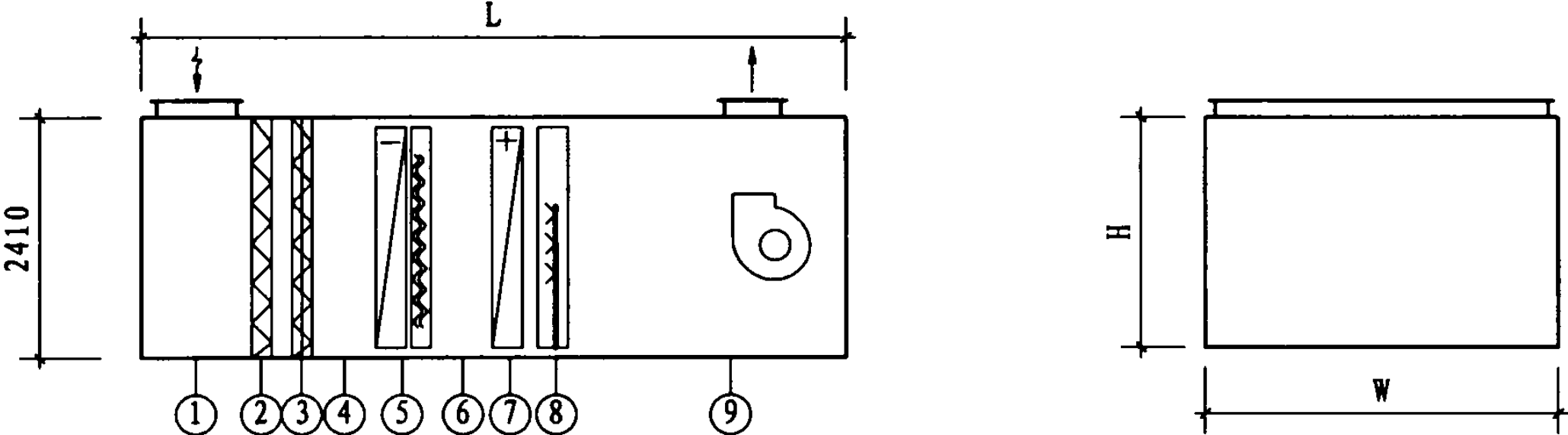
示例十三：机房内设一台60000m³/h风量卧式空气处理机（单风机）
