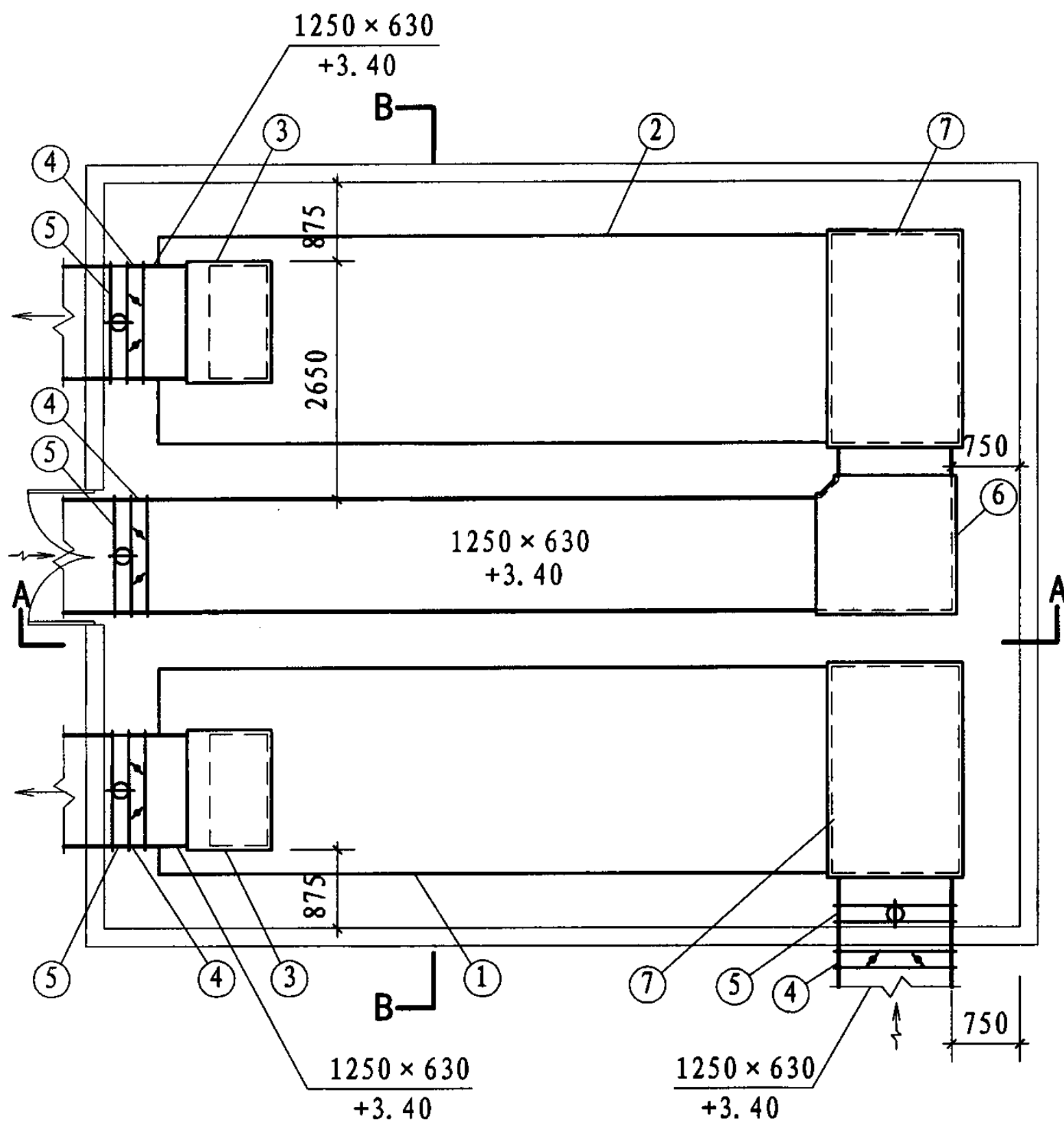
送风、回风风管平面图
