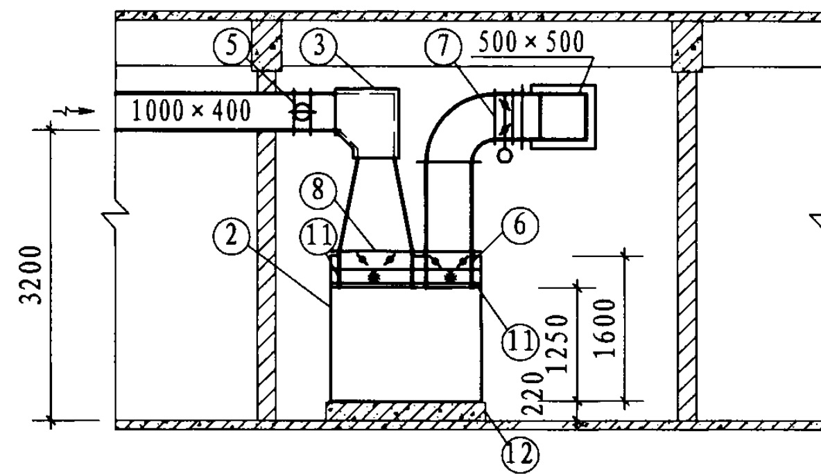
B-B
