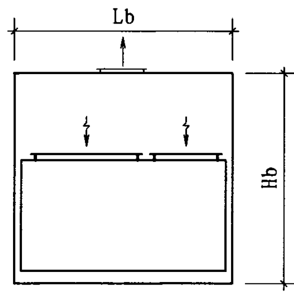
空气处理机组段形式B（带加湿器）
