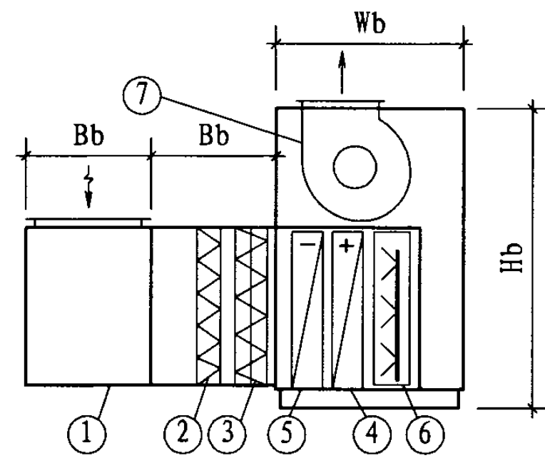
空气处理机组段形式B（带加湿器）
