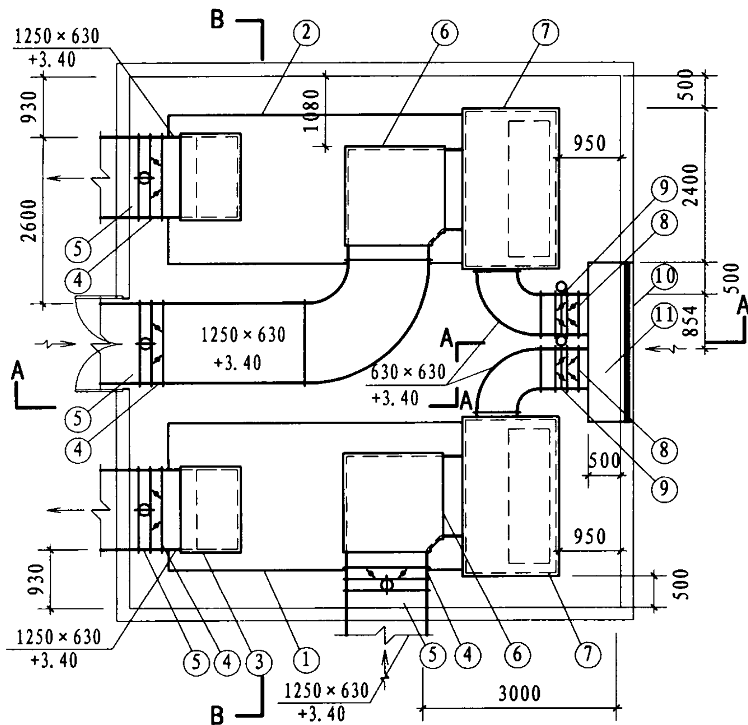
风管平面图
