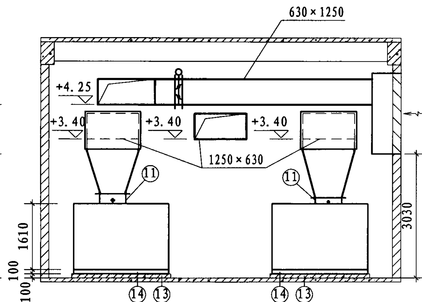
B-B
