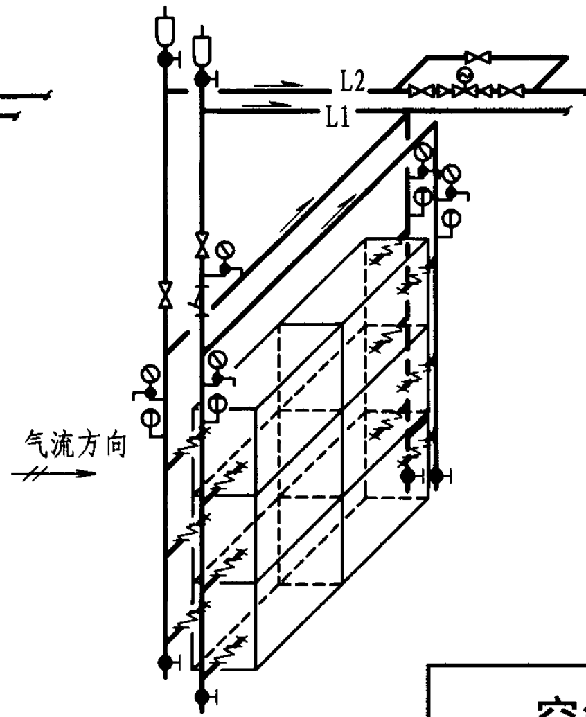
六台冷却器接管示意图
