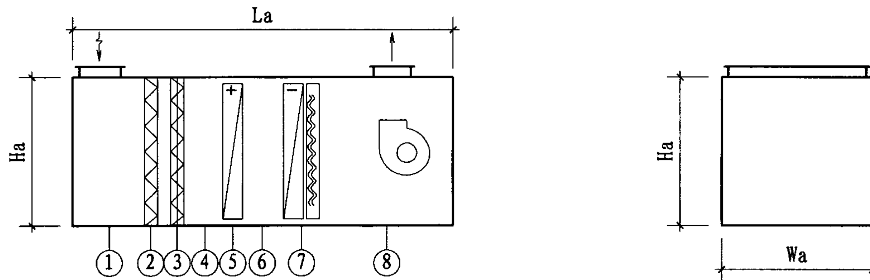
空气处理机A组段形式
