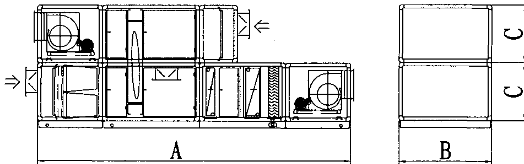
卧式标准转轮式带旁通热回收机组
