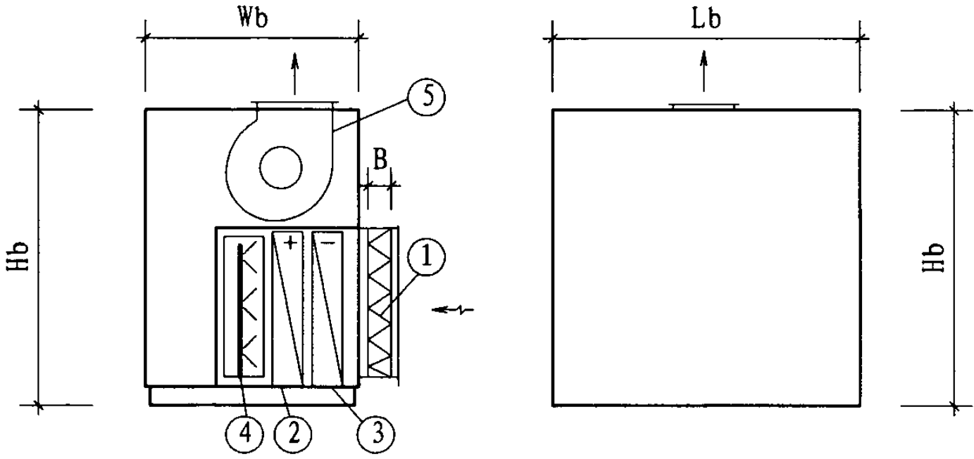
空气处理机组段形式B（带加湿器）
