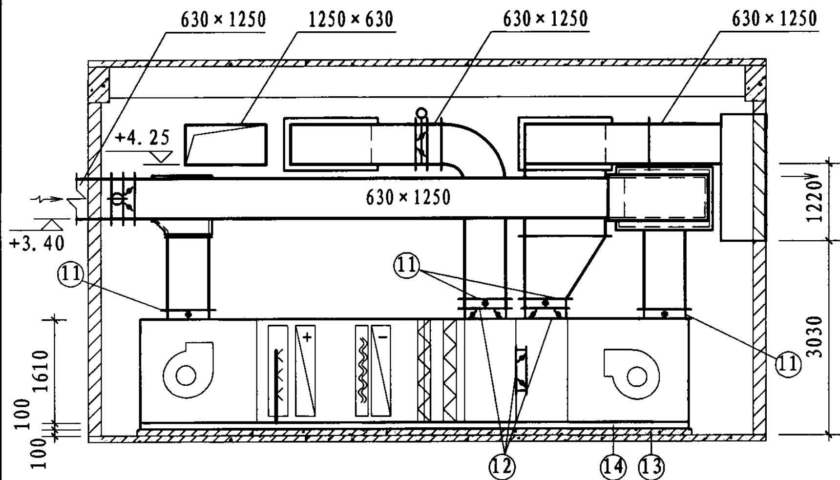
A-A
