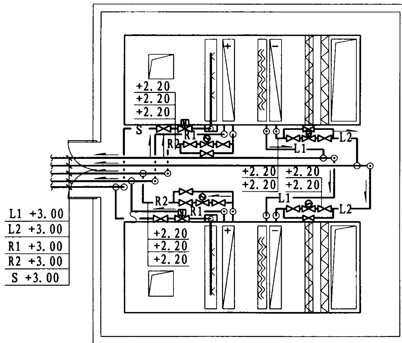
水管平面图
