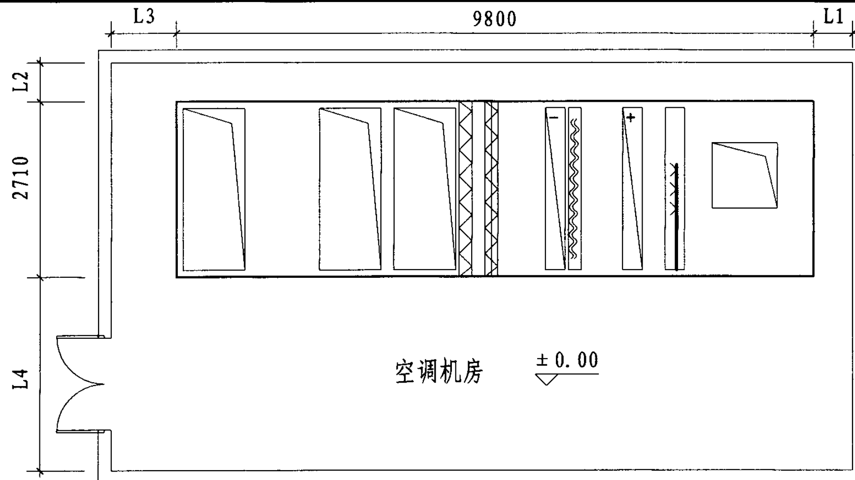
设备平面布置图
