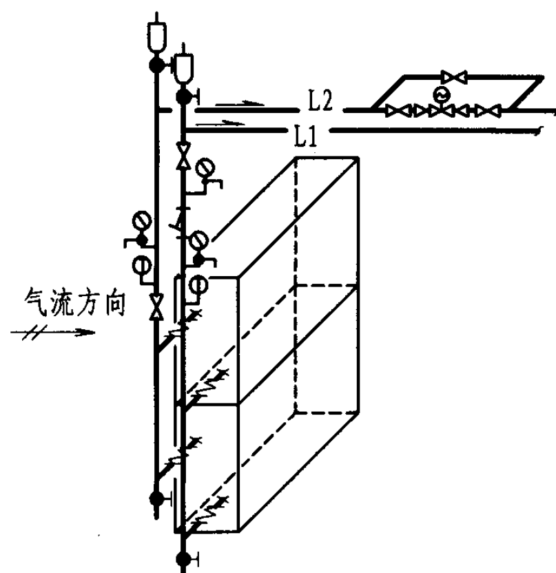
两台冷却器接管示意图
