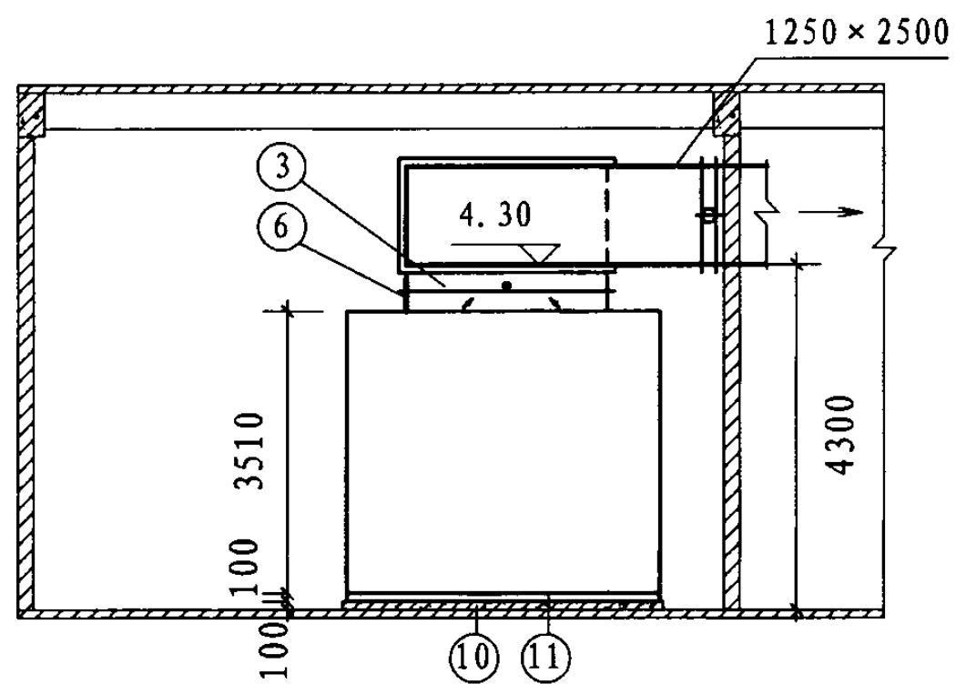
B-B
