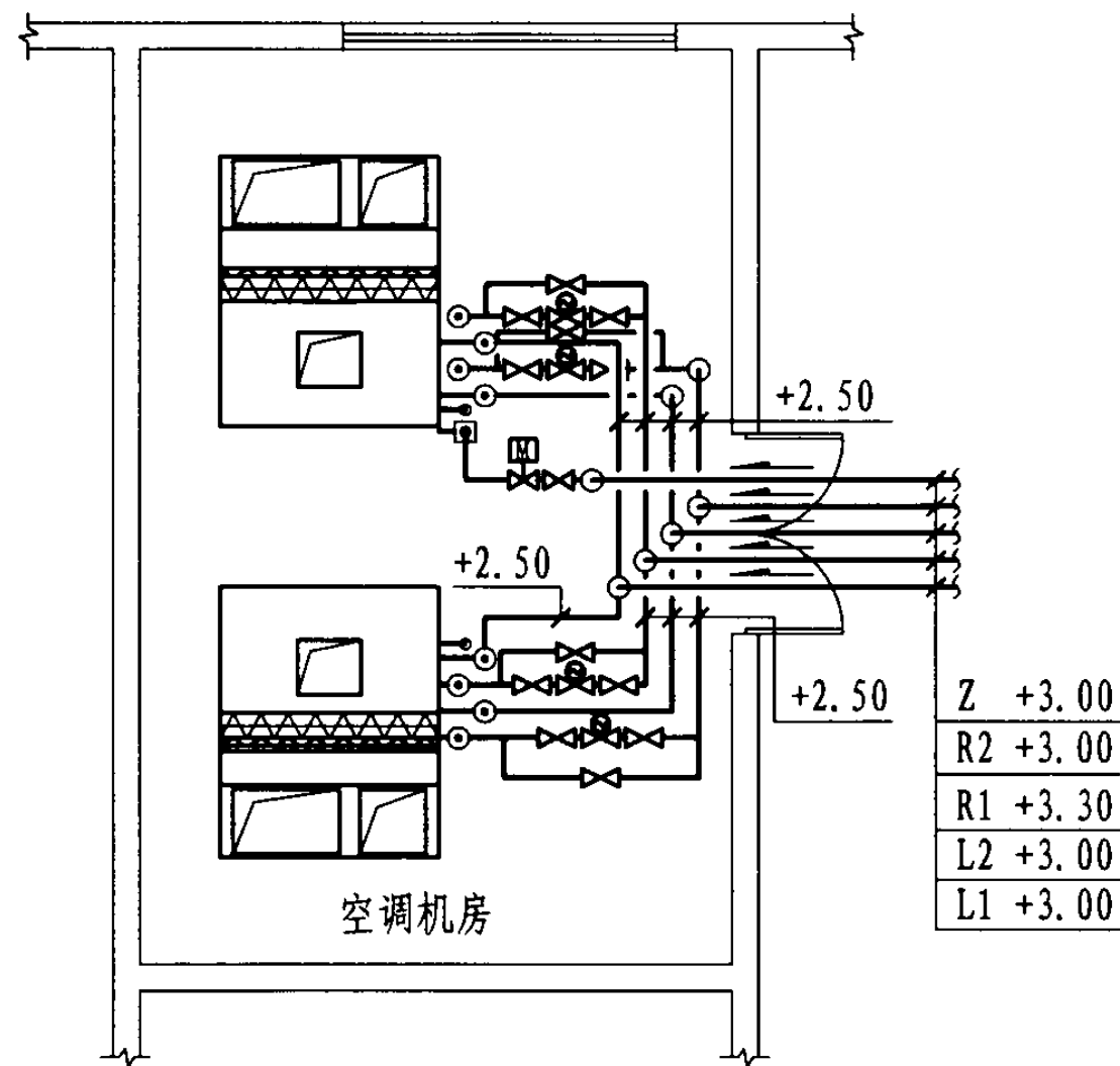
水管平面图
