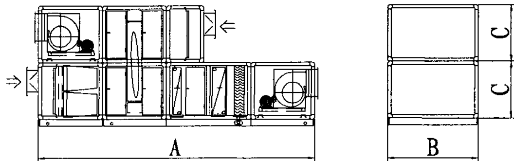
卧式标准转轮式热回收机组
