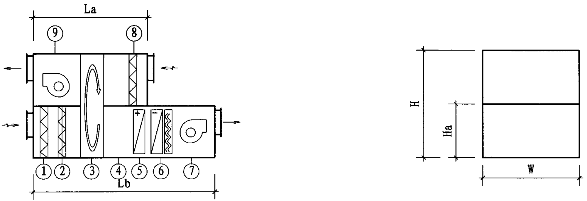
示例七：机房内设一台20000m³/h风量卧式空气处理机（带全热回收）
