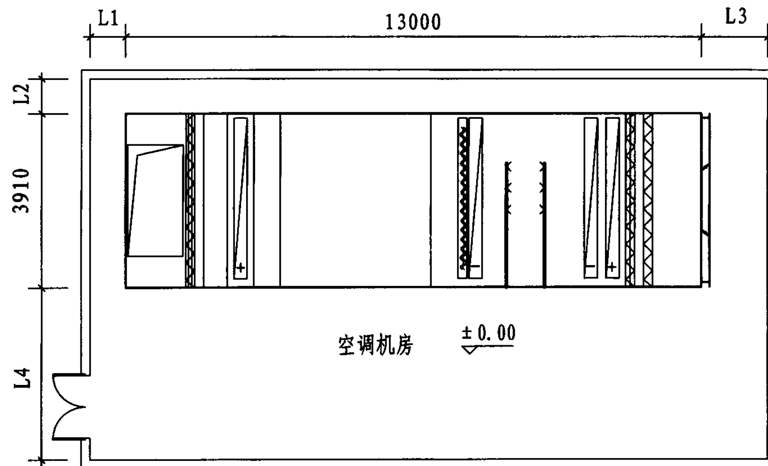
设备平面布置图
