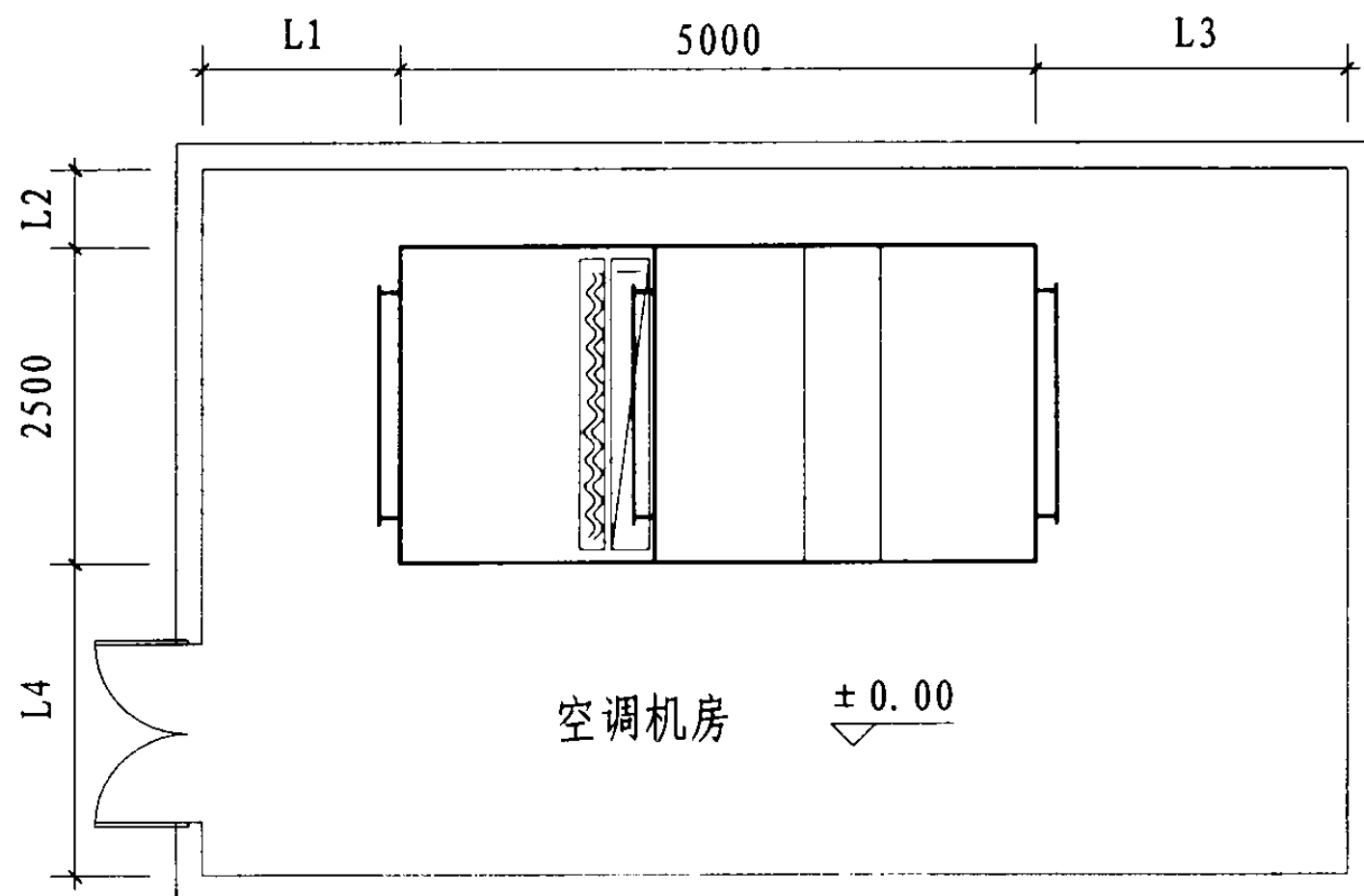
设备平面布置图
