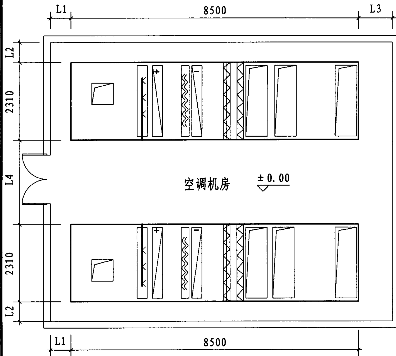
设备布置图
