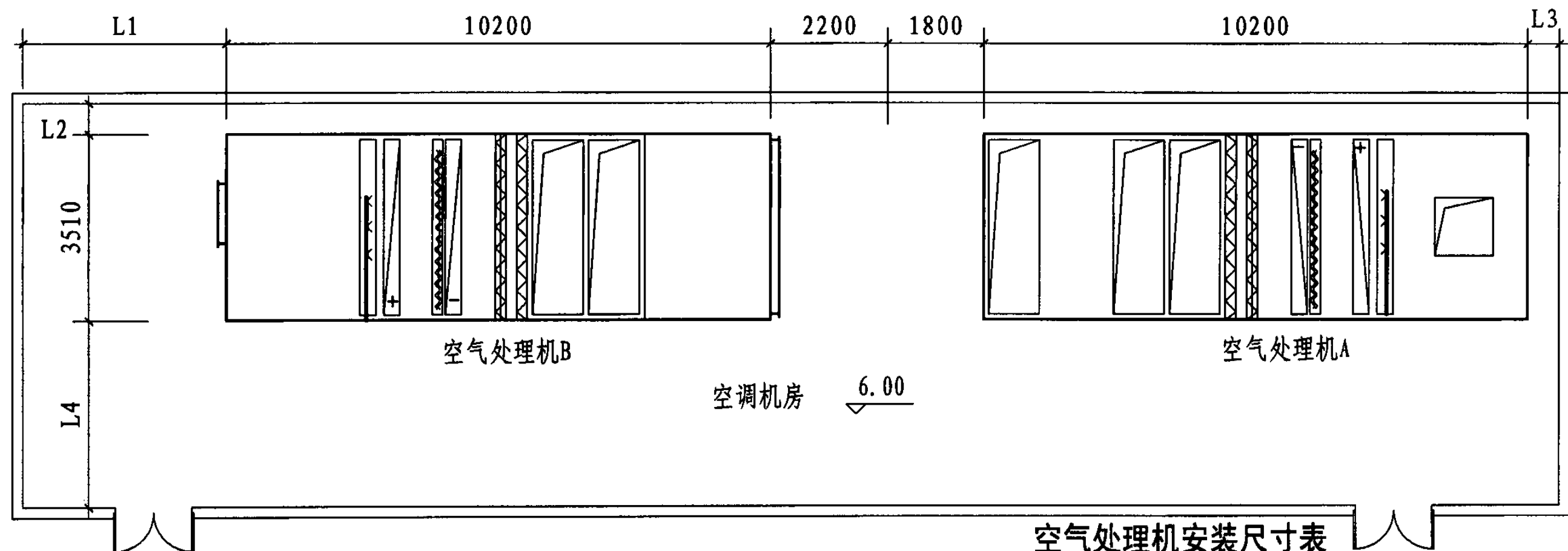
设备布置图
