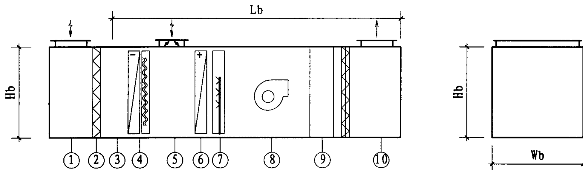
空气处理机B组段形式
