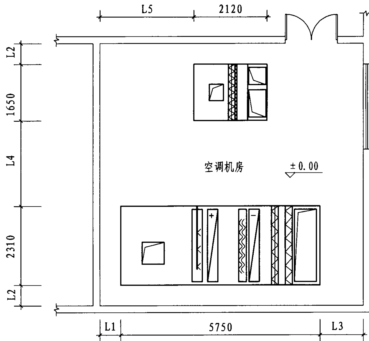
设备布置图
