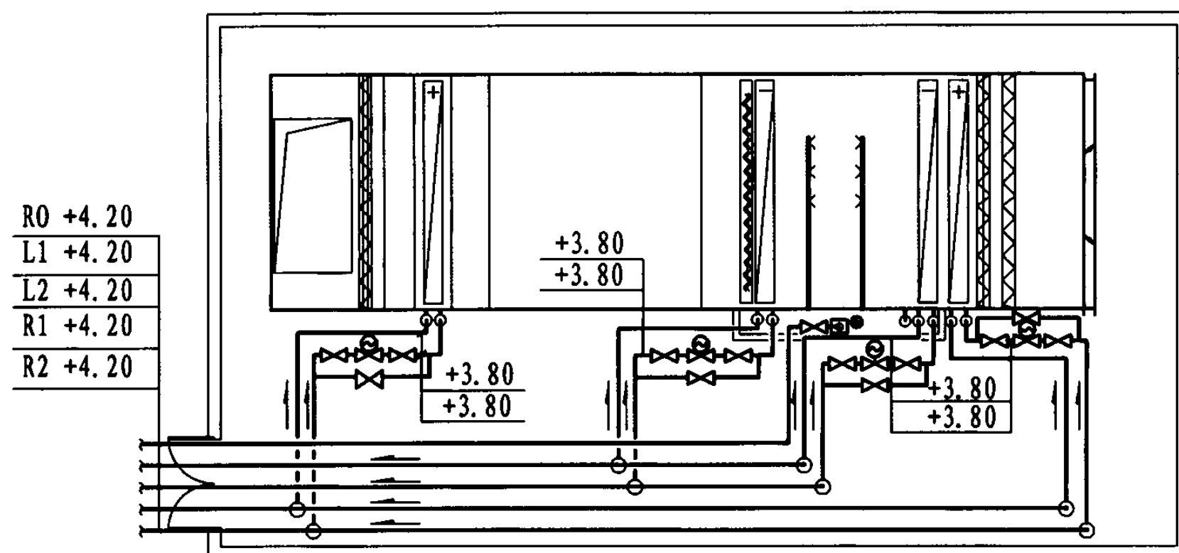
水管平面图
