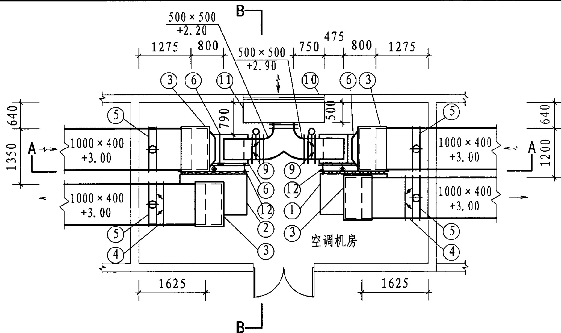
风管平面图
