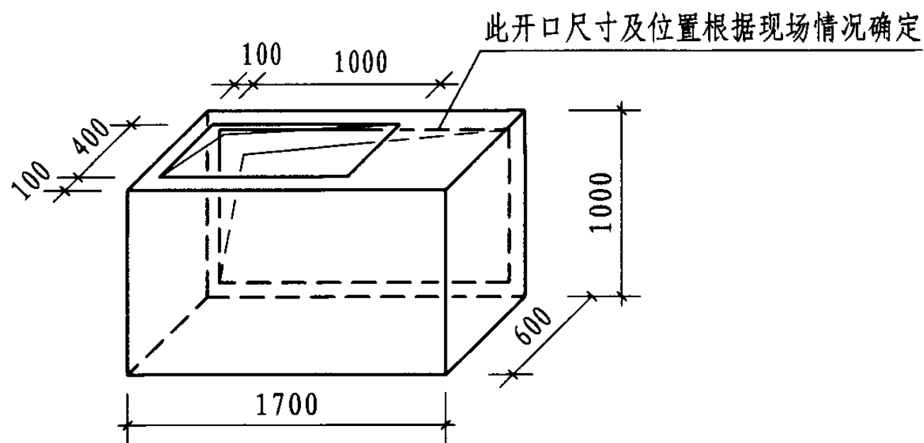
联箱详图
