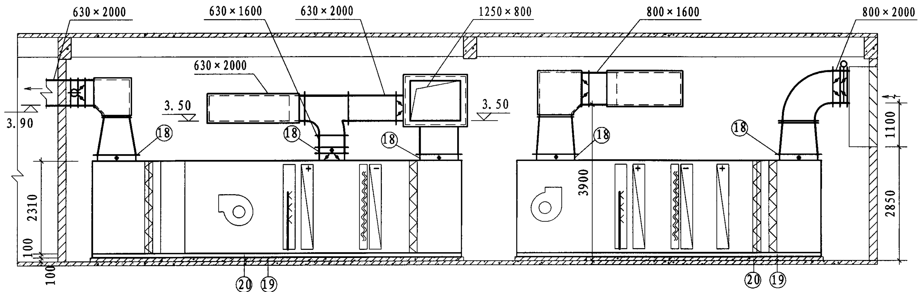
A-A
