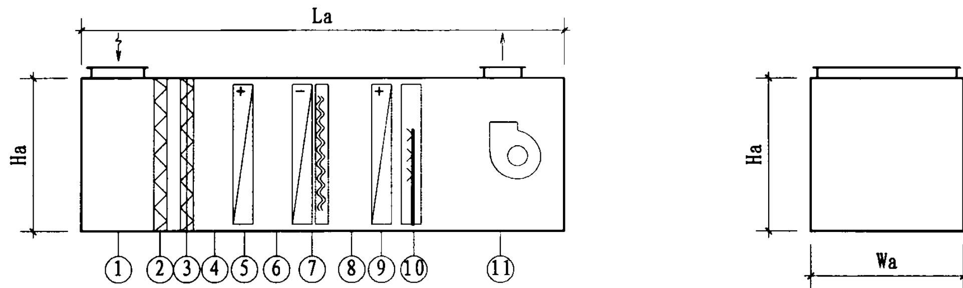
空气处理机A组段形式
