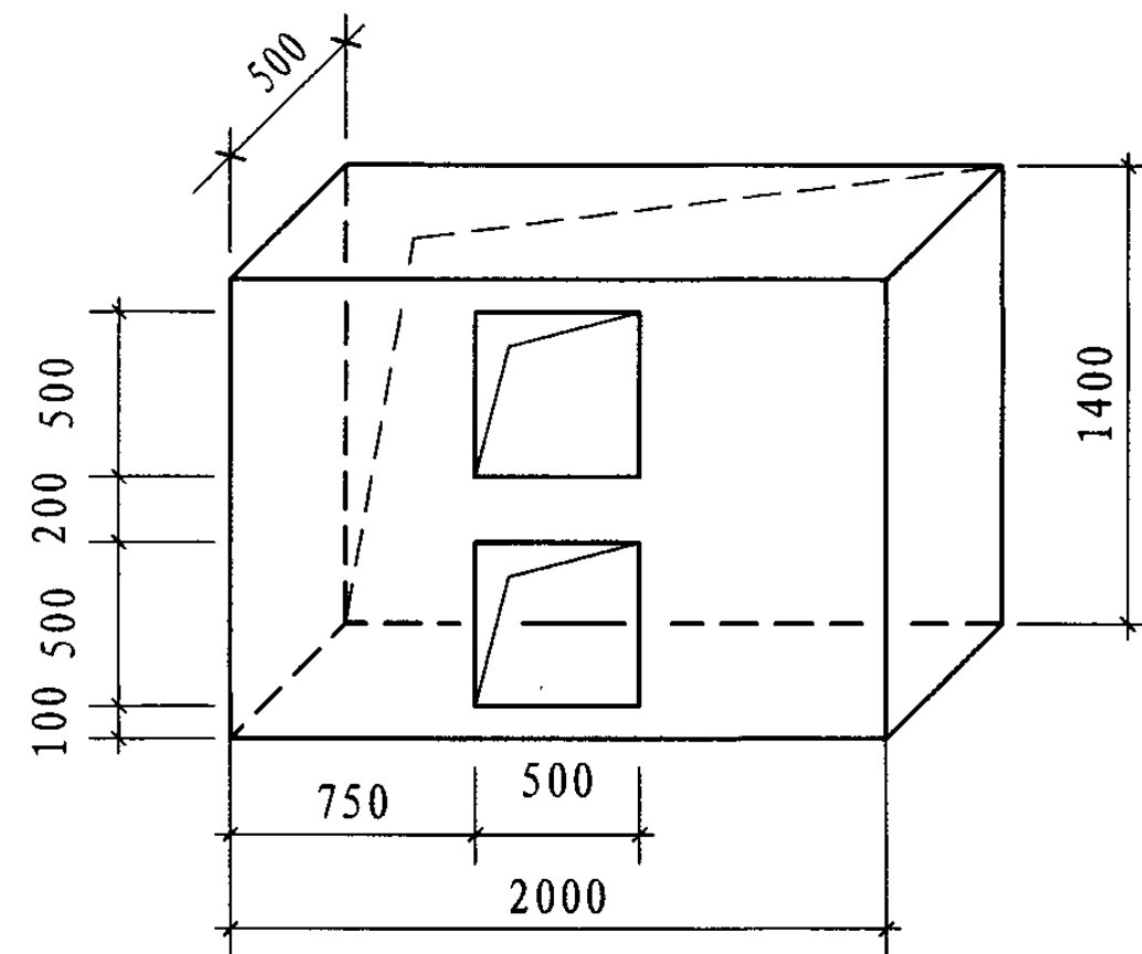
新风百叶联箱示意图
