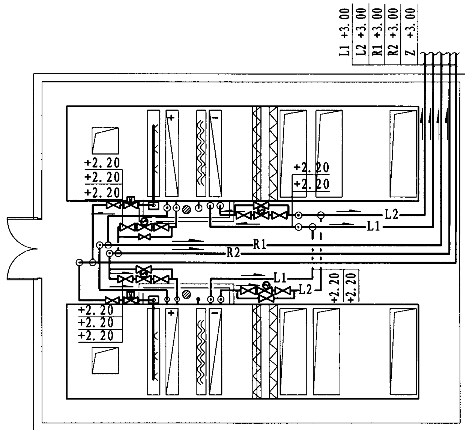
水管平面图
