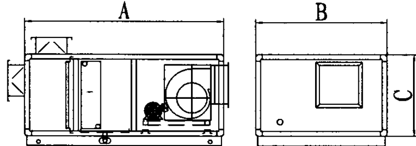
卧式标准机组二
