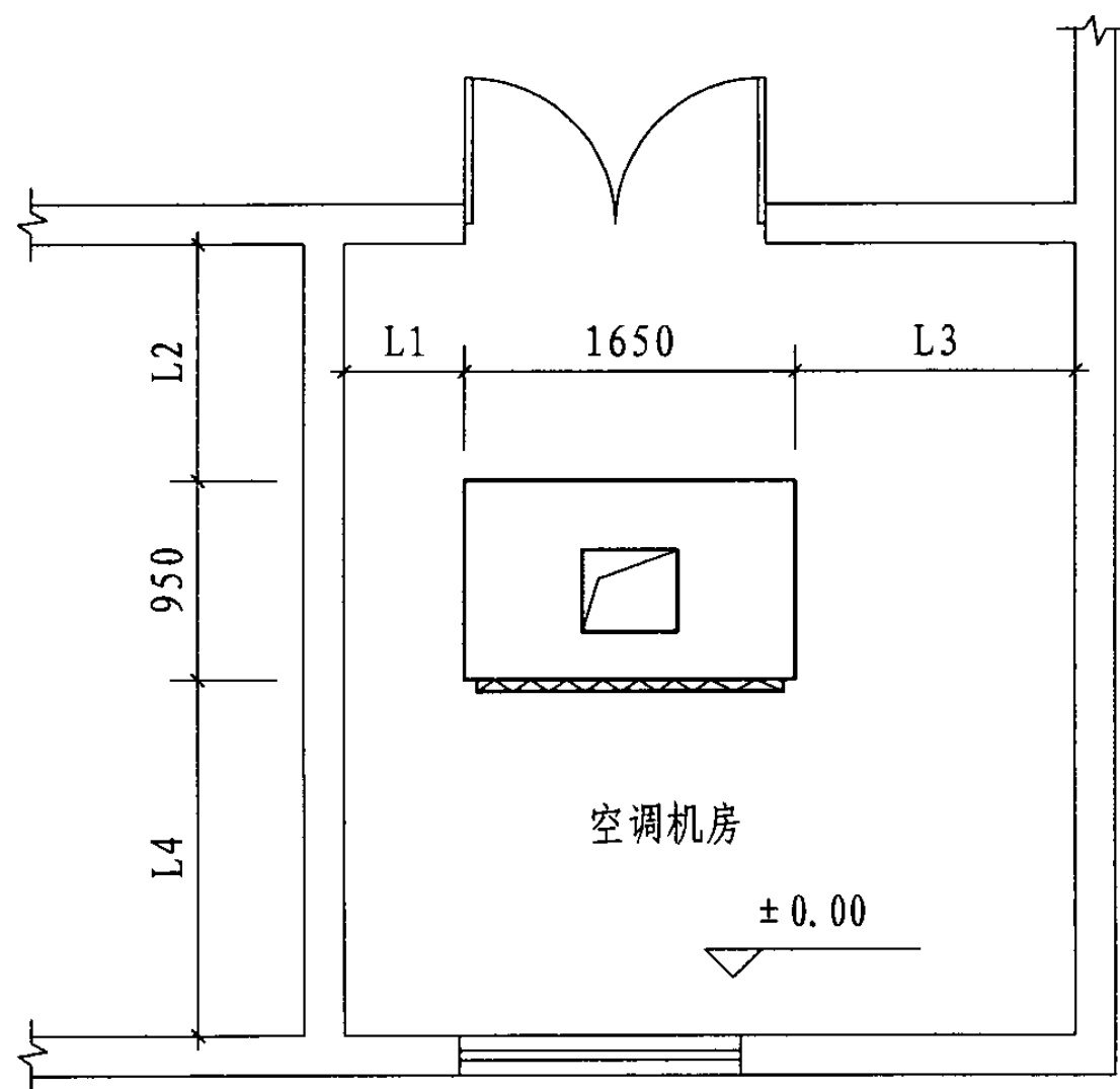
设备布置图
