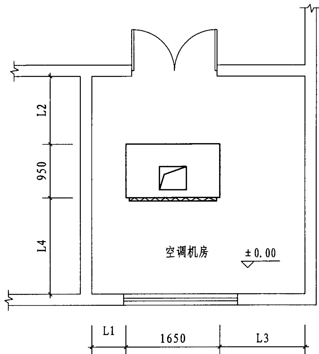
设备布置图
