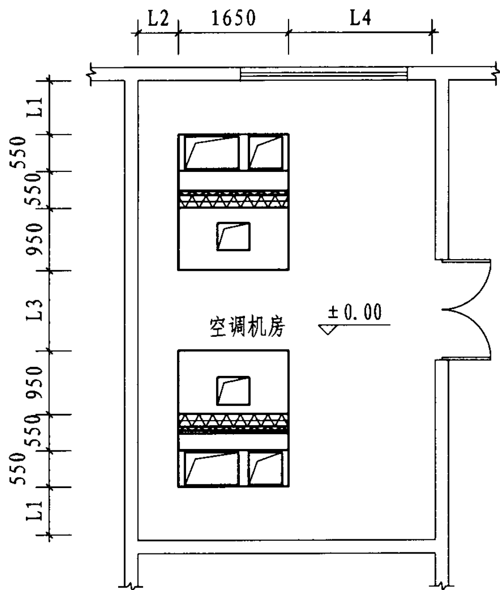
设备布置图
