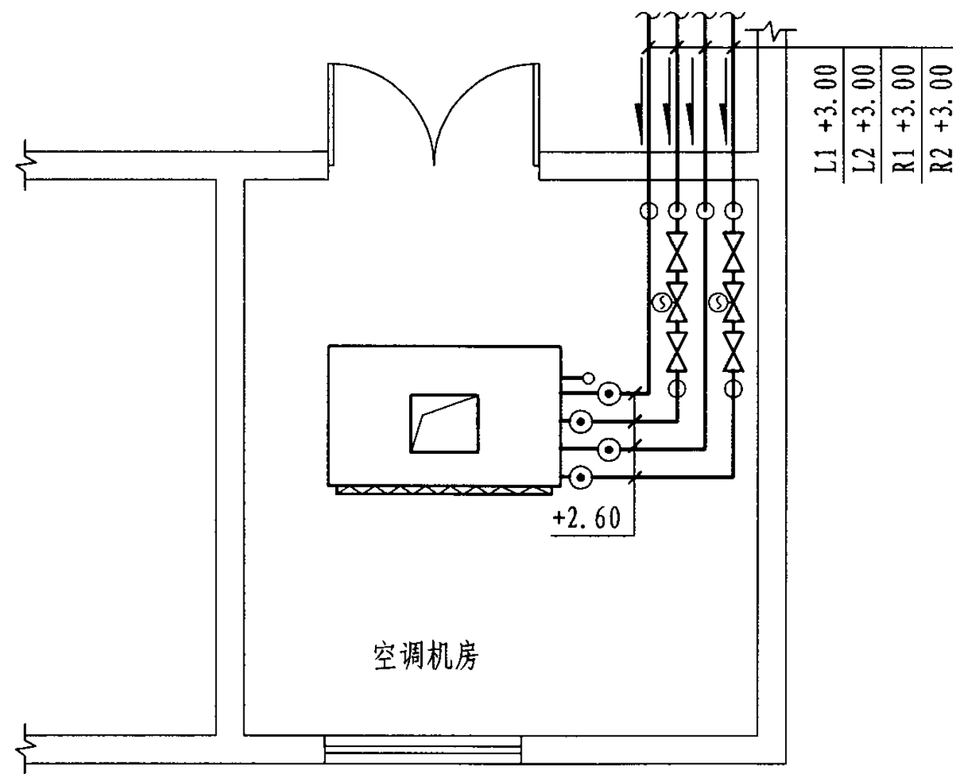
水管平面图
