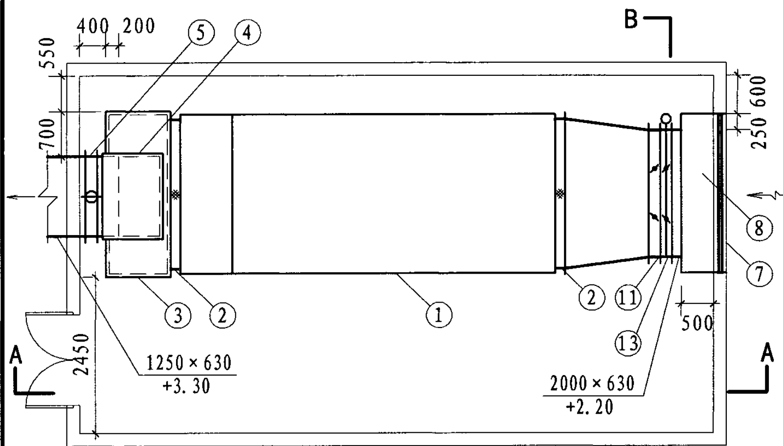
新风风管平面图
