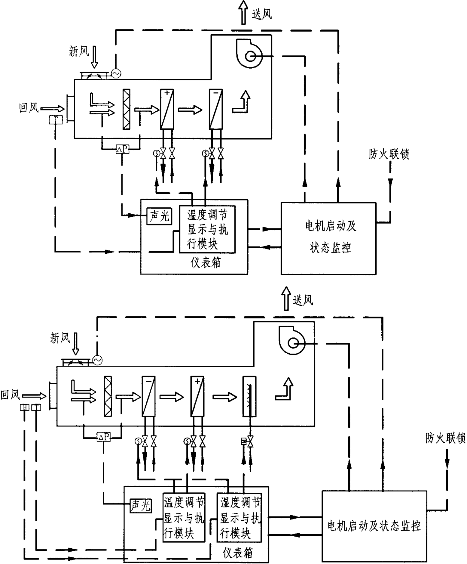
示例二空调原理图
