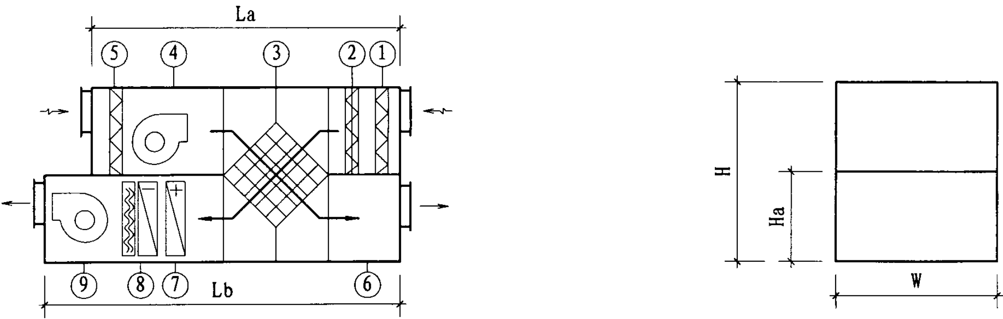
示例六：机房内设一台20000m³/h风量卧式空气处理机（带显热回收）
