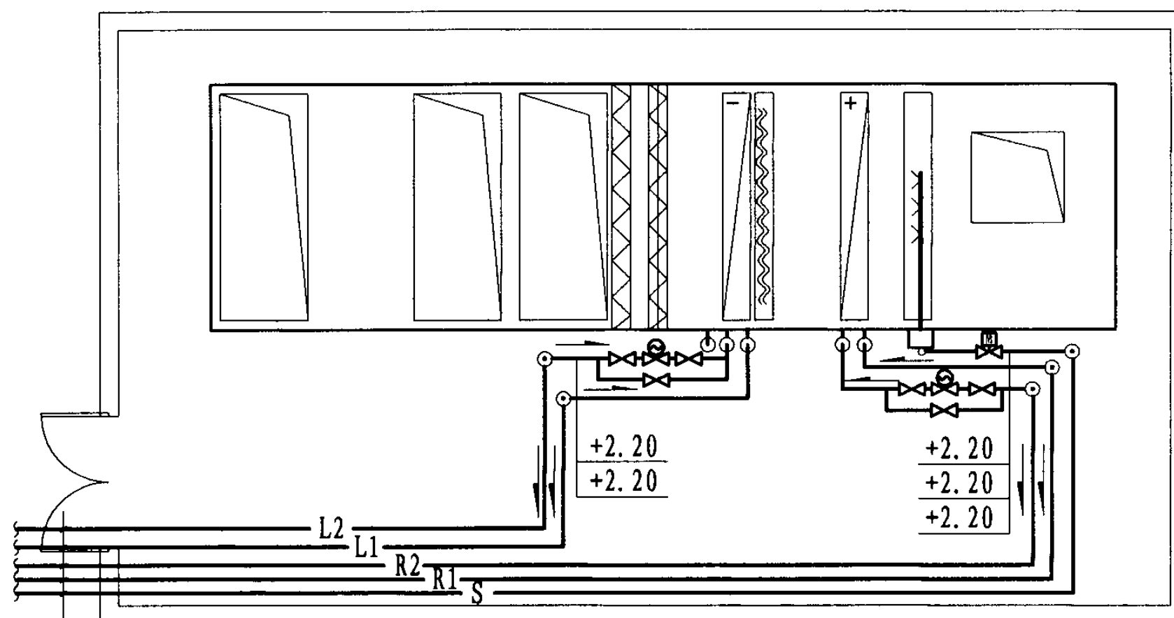
水管平面图
