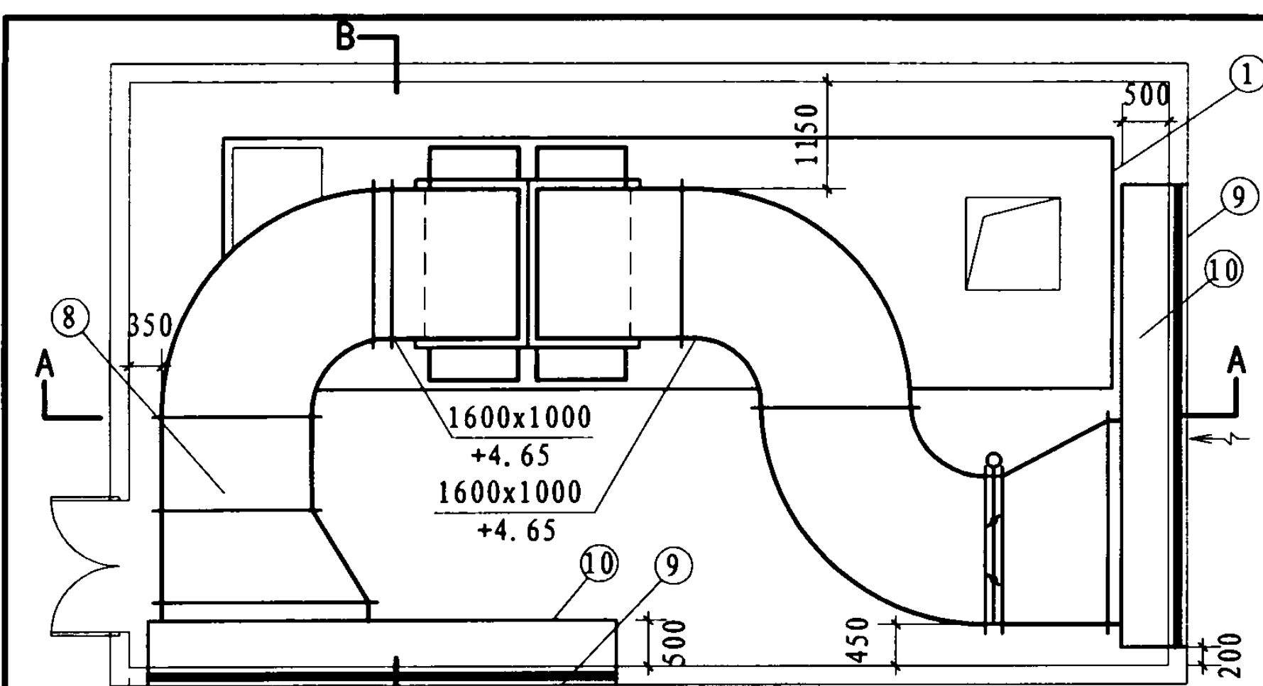
新风、排风风管平面图
