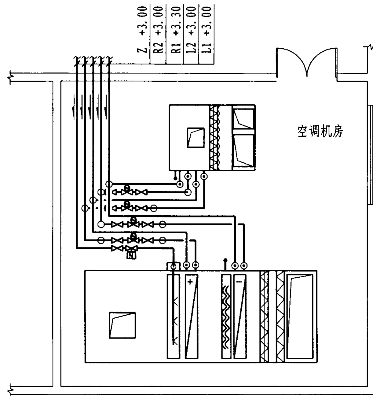
水管平面图
