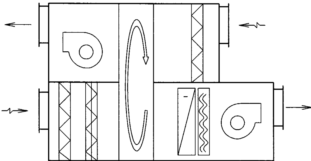
转轮式能量回收空气处理机组
