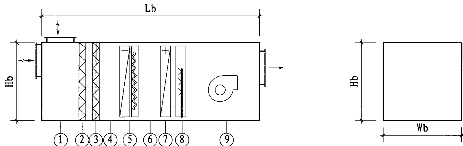
空气处理机B组段形式
