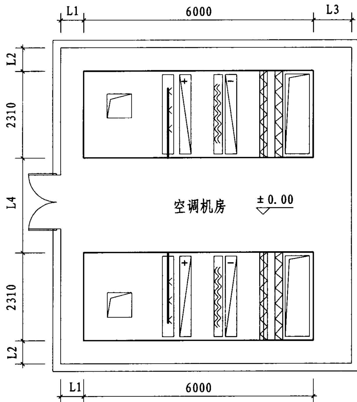
设备布置图
