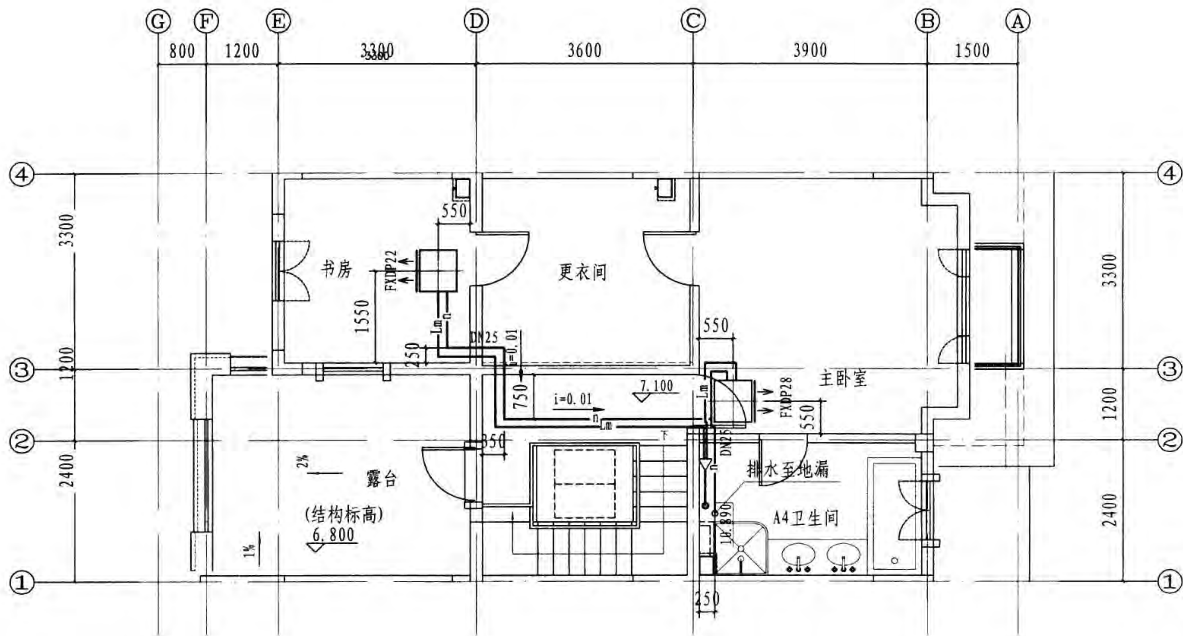
三层空调平面图
