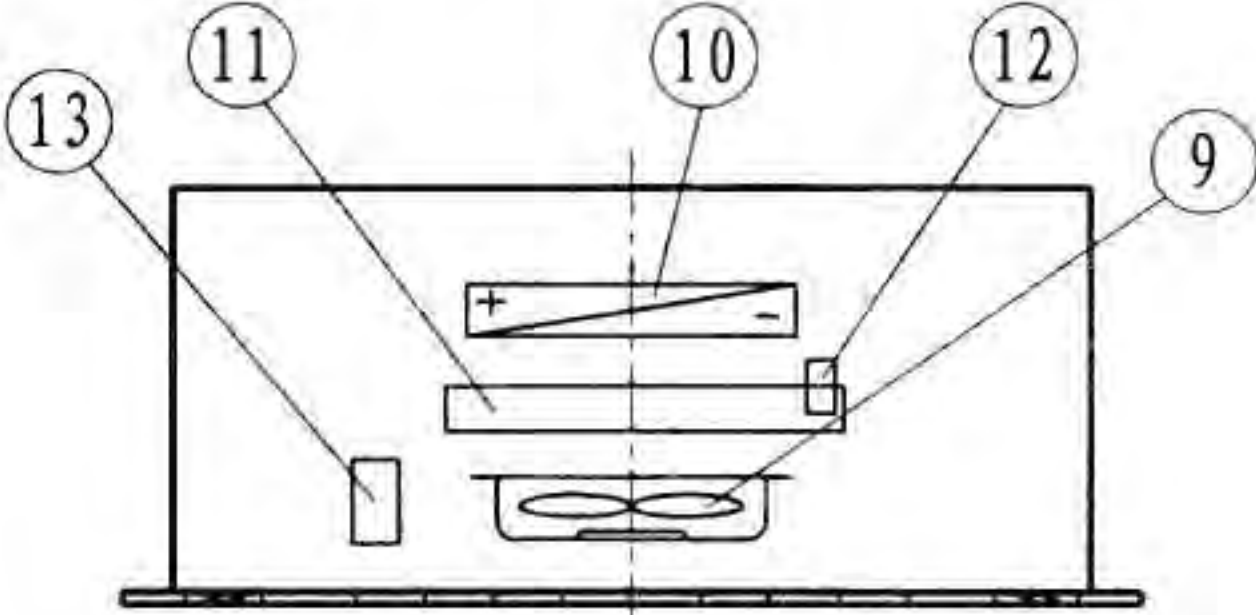
I - I 剖视图
