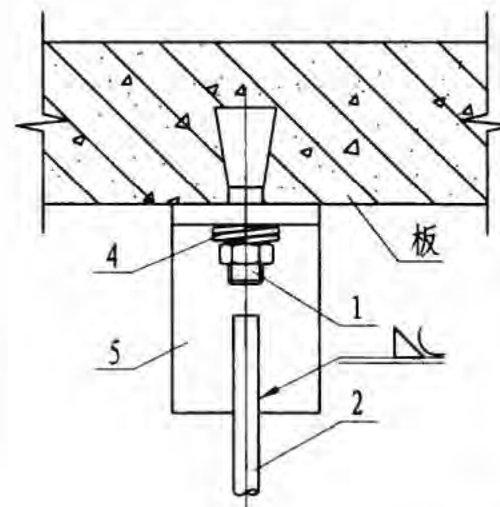
胀锚螺栓生根 V
