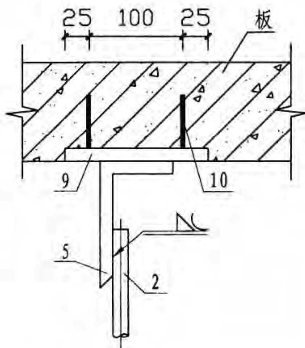
预埋件生根 II
