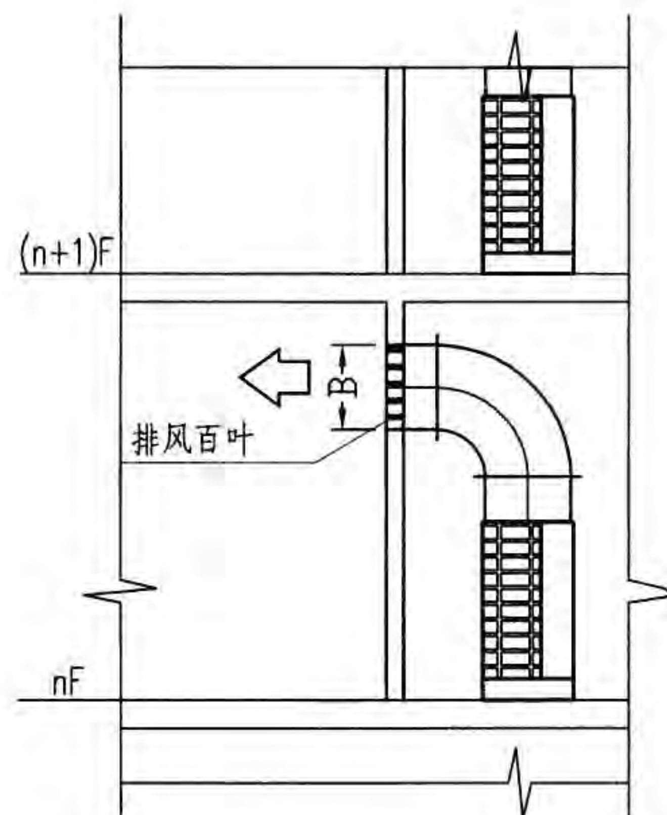
III-III剖面图
