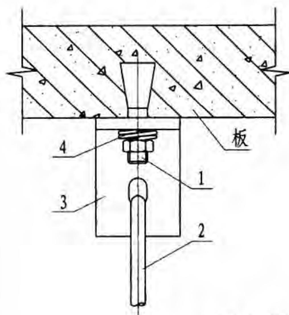
胀锚螺栓生根 IV
