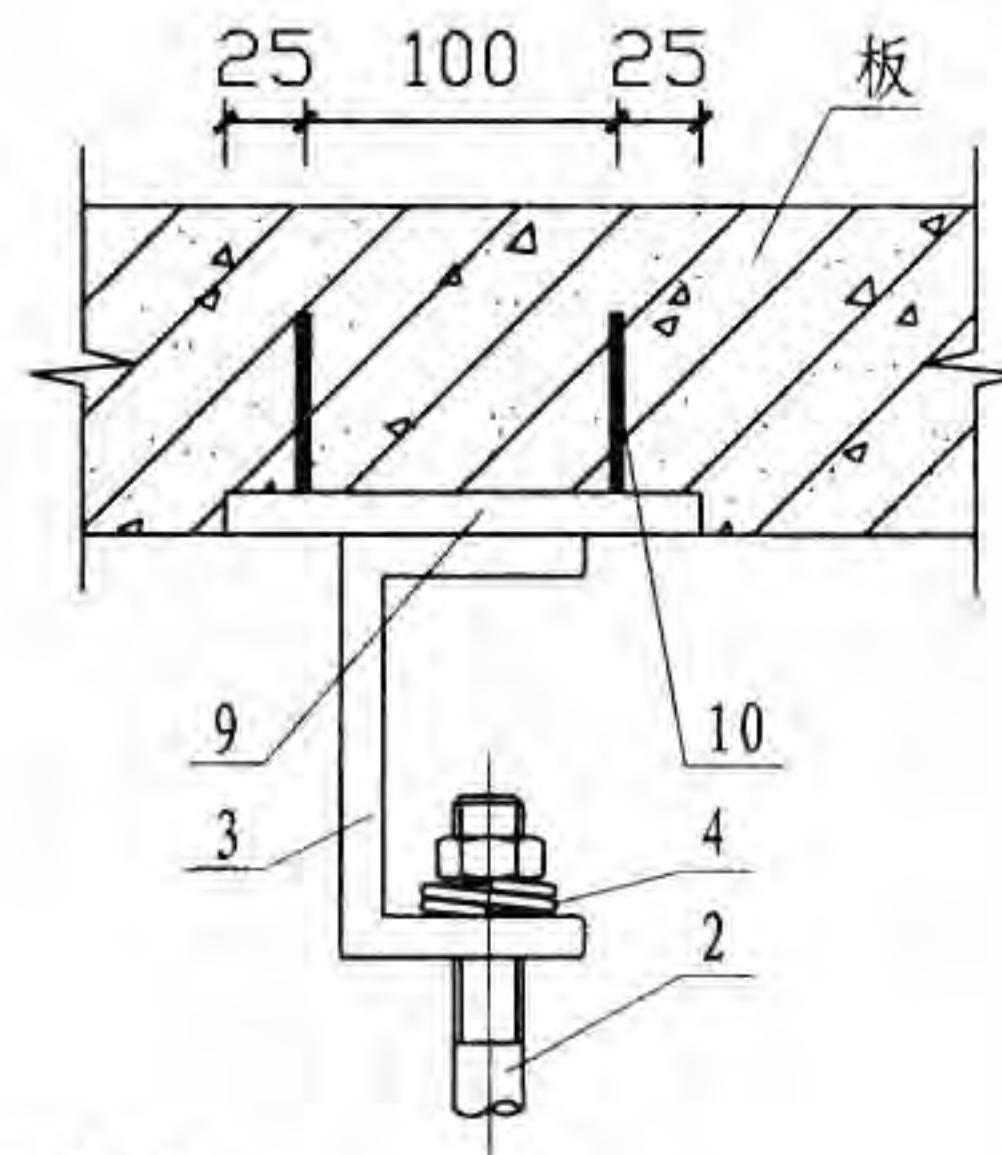
预埋件生根 I
