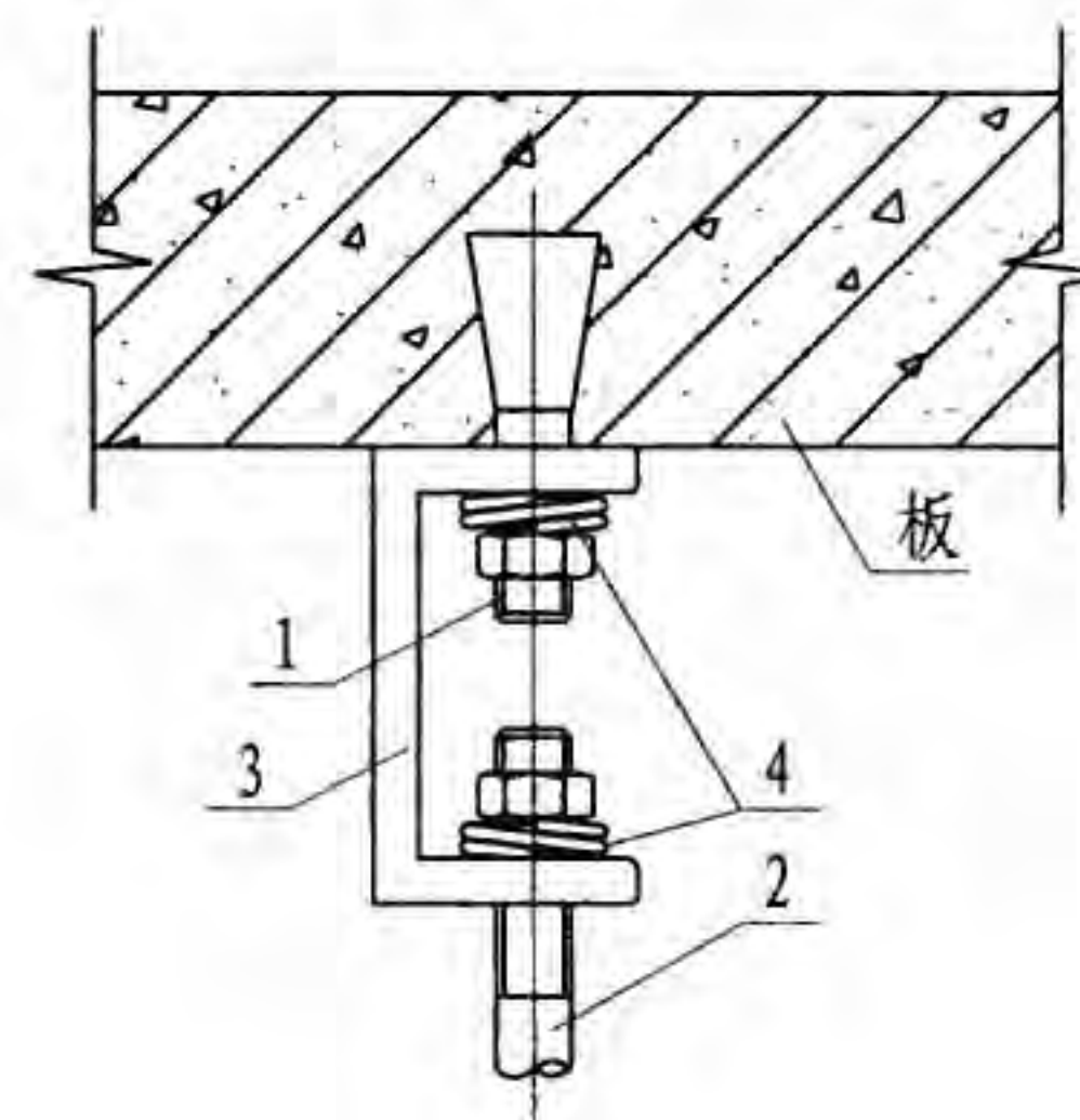
胀锚螺栓生根 III
