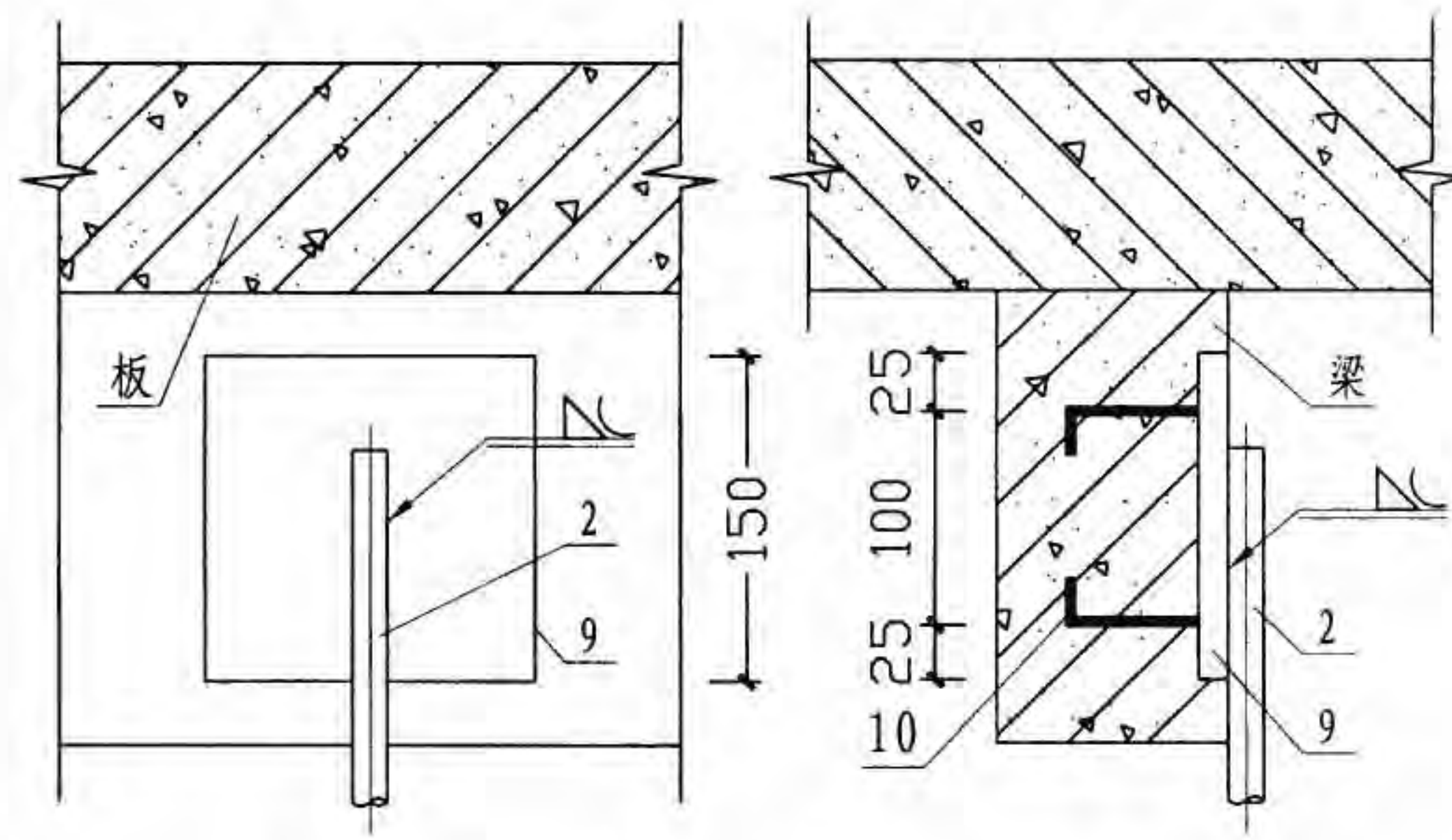
预埋件生根 III
