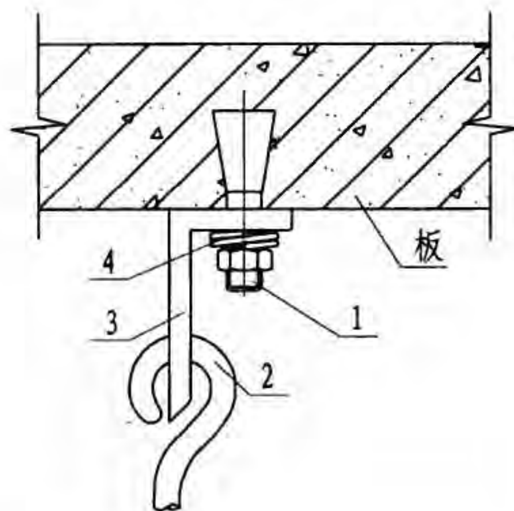
胀锚螺栓生根 IV
