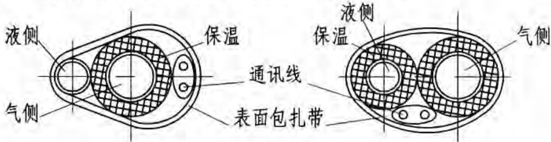
附图1 气液侧间隔热做法
