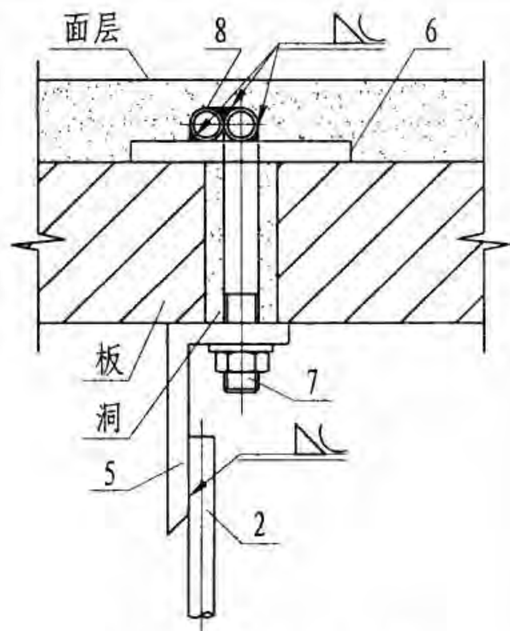
穿楼板螺栓生根 IV
