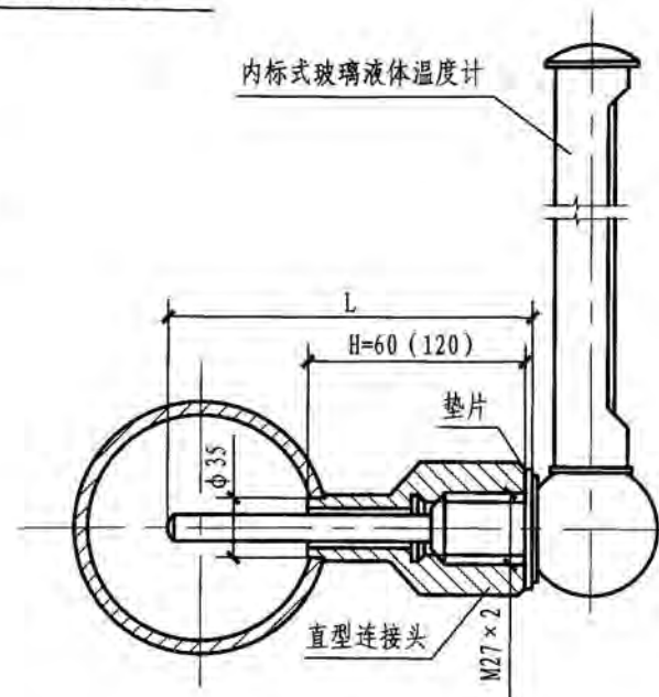
90°角型温度计安装图
