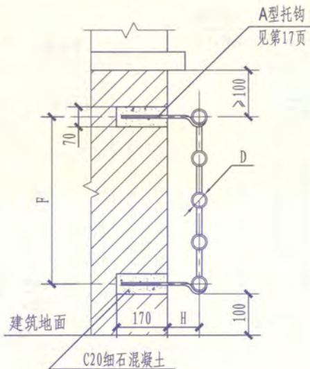
热水排管散热器砖墙上安装
