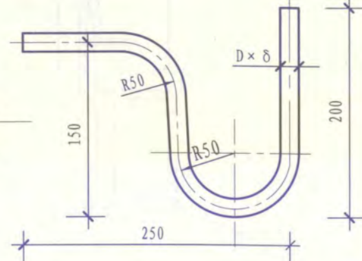
冷凝弯
