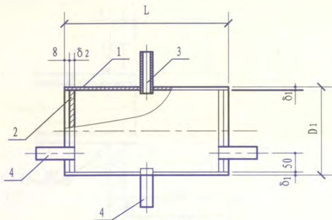
卧式集气罐
