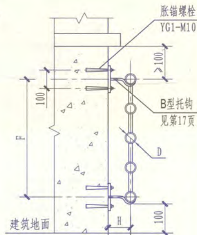
热水排管散热器混凝土墙上安装
