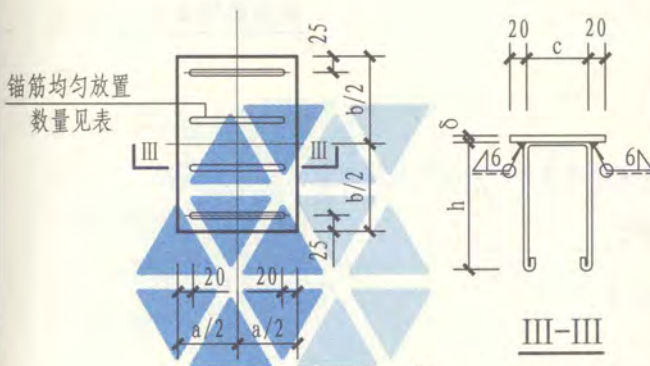
底板
