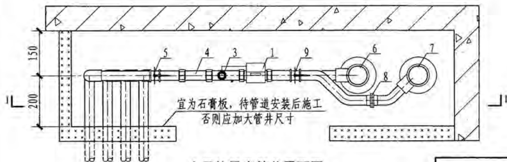
户用热量表管井平面图
