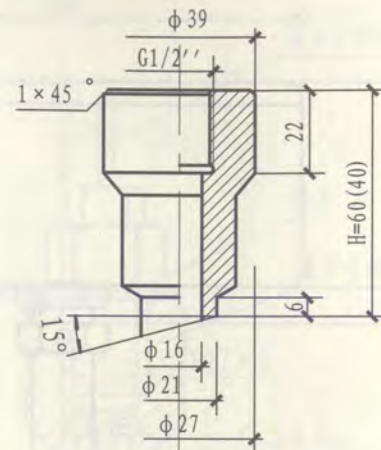
15°角接头
