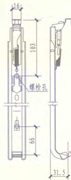
弹簧支架
