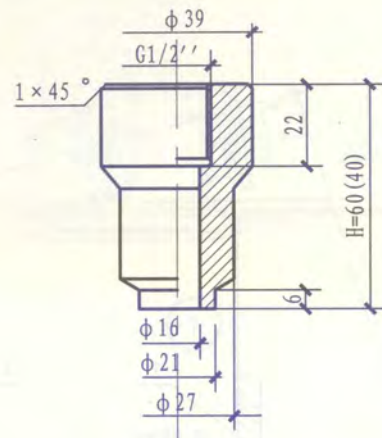
直型连接头
