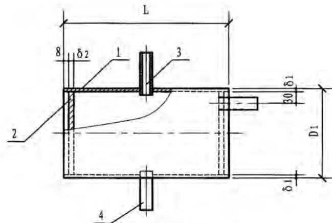
卧式集气罐
